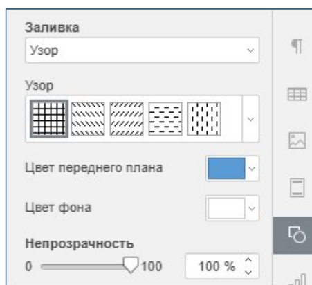
Рисунок 120 – Узор
