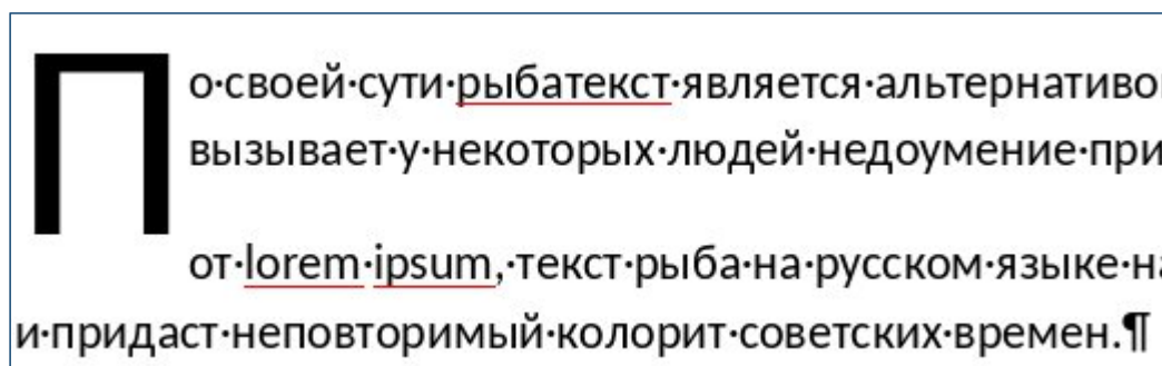
Рисунок 88 – Пример буквицы
