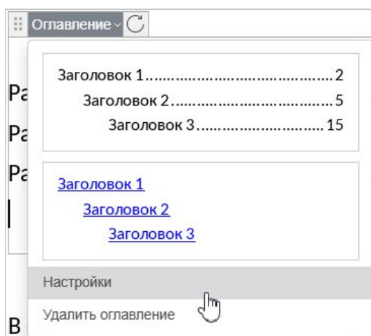
Рисунок 175 – Настройки оглавления
