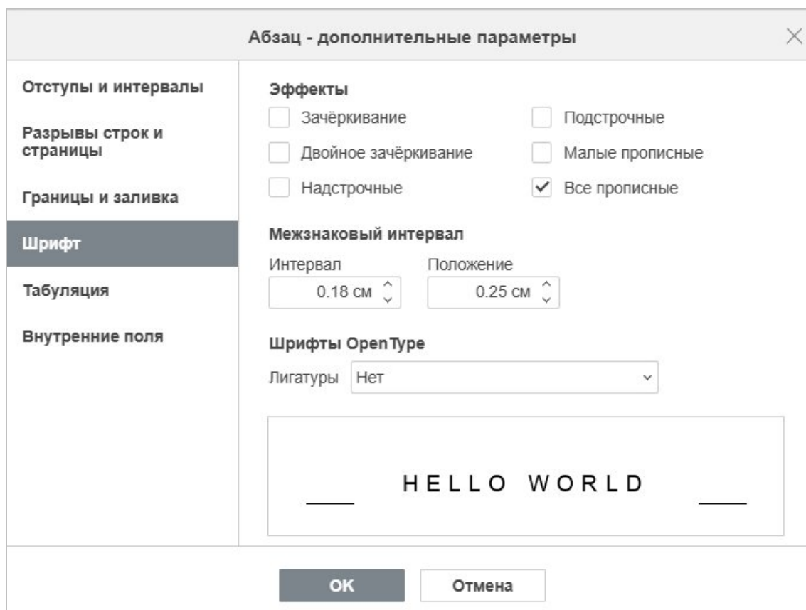
Рисунок 83 – Вкладка «Шрифт»
