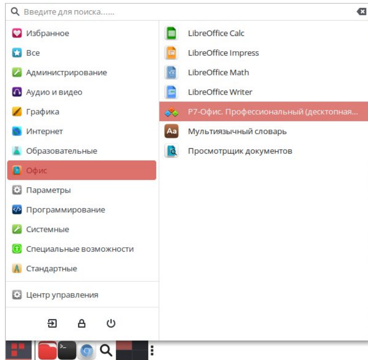
Рисунок 4 – Запуск программы
