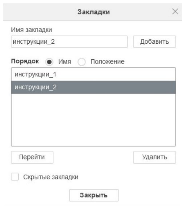
Рисунок 64 – Выбор закладки
