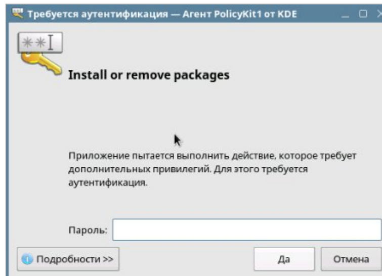
Рисунок 7 – Ввод пароля
