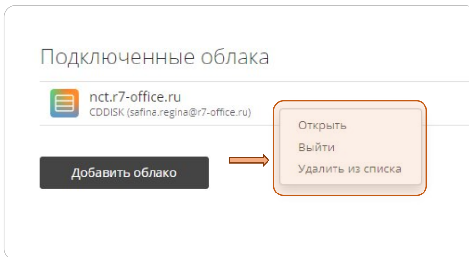
Рисунок 227 – Удаление облака
