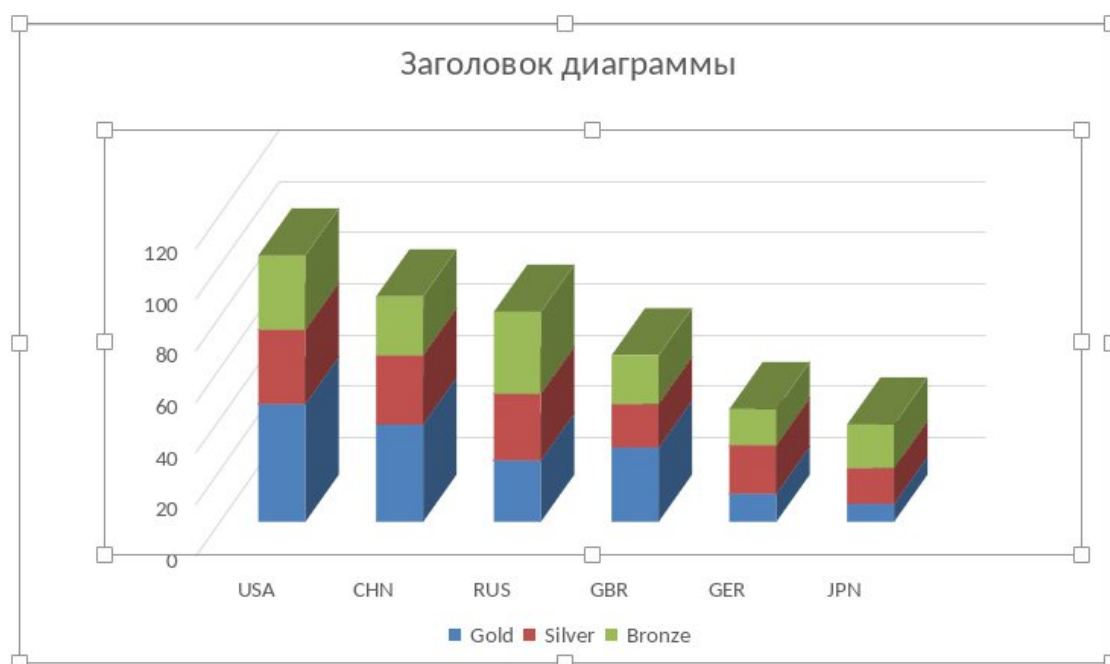
Рисунок 141 – 3D-диаграмма
