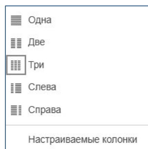
Рисунок 44 – Колонки
