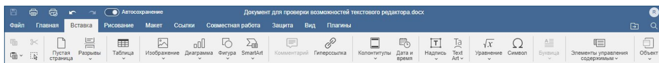
Рисунок 25 – Вкладка «Вставка»
