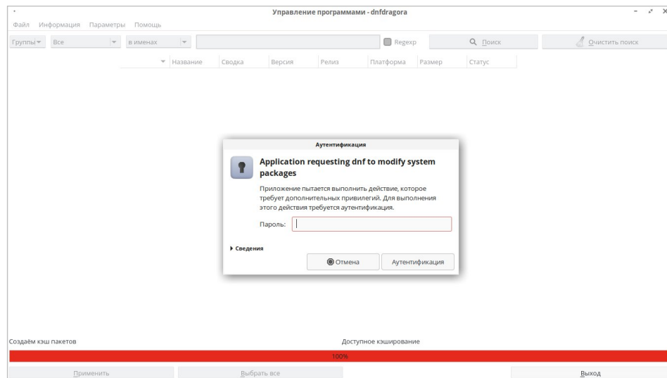
Рисунок 2 – Ввод пароля
