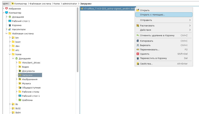
Рисунок 5 – Запуск установки
