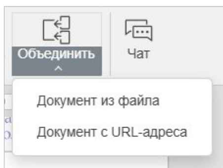
Рисунок 201 – Инструмент «Объединить»
