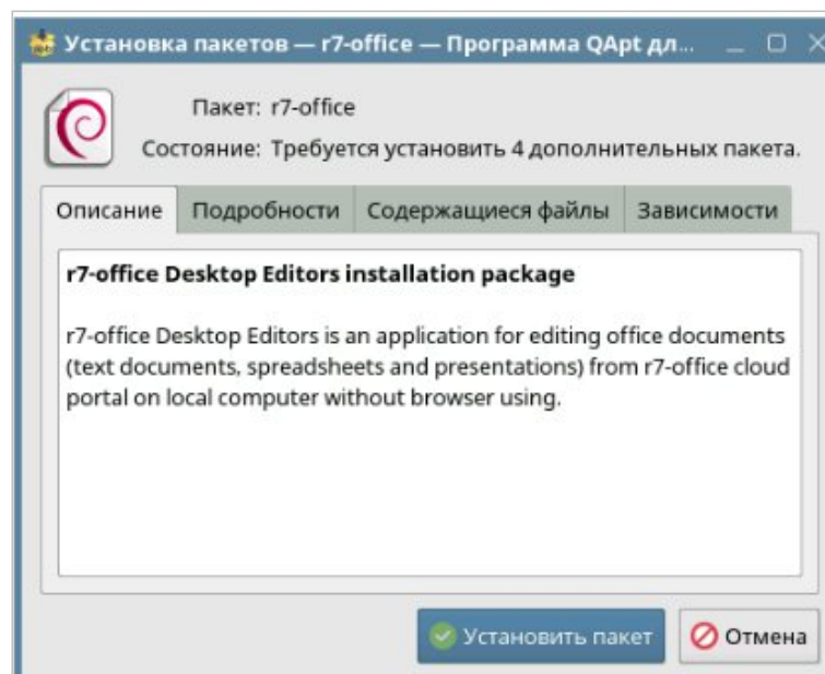
Рисунок 6 – Окно установки
