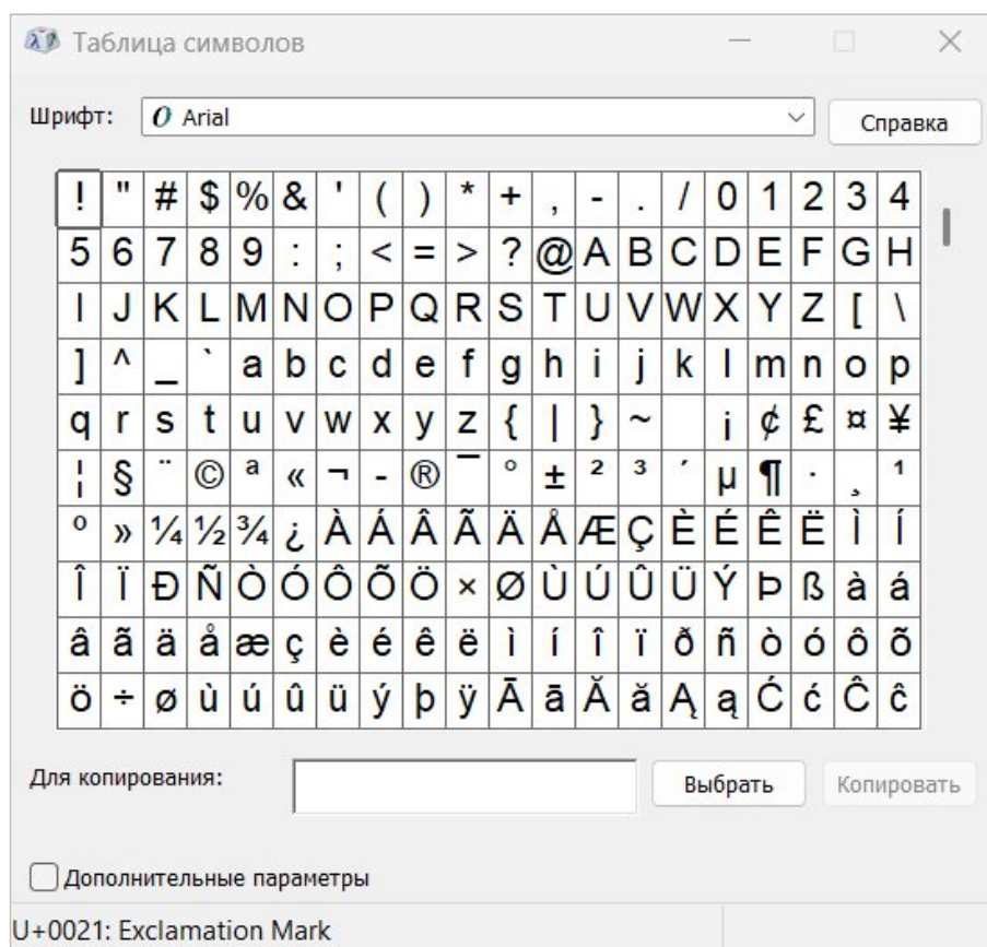
Рисунок 158 – Таблица символов
