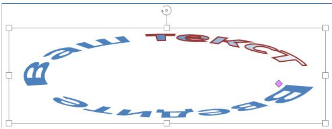
Рисунок 152 – Трансформации текста
