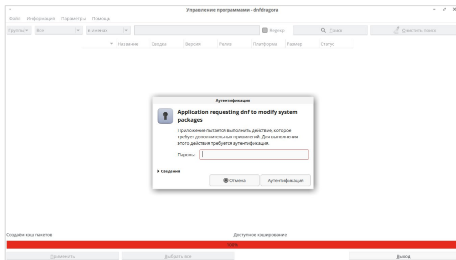
Рисунок 2 – Ввод пароля
