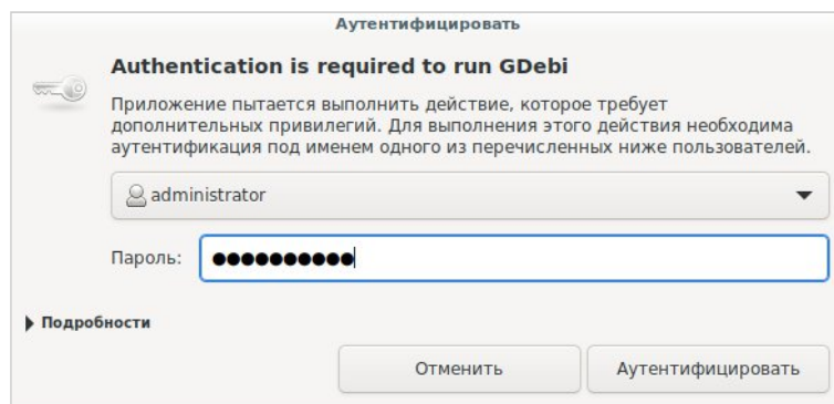
Рисунок 11 – ввод пароля
