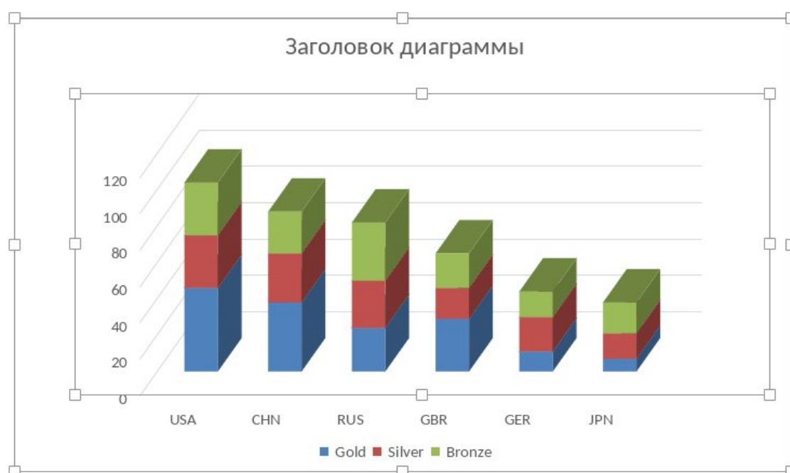
Рисунок 98 – 3D-диаграмма
