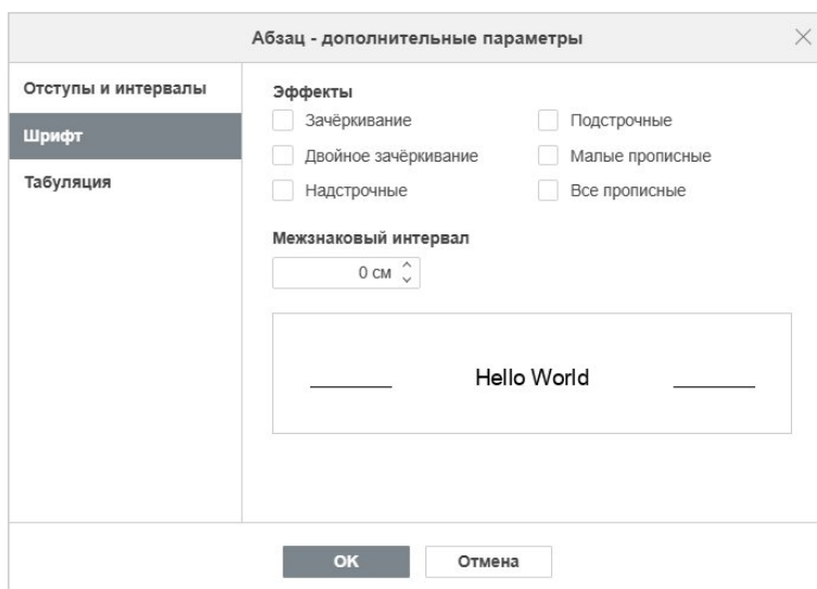
Рисунок 59 – Вкладка «Шрифт»
