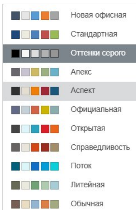
Рисунок 43 – Цветовые схемы
