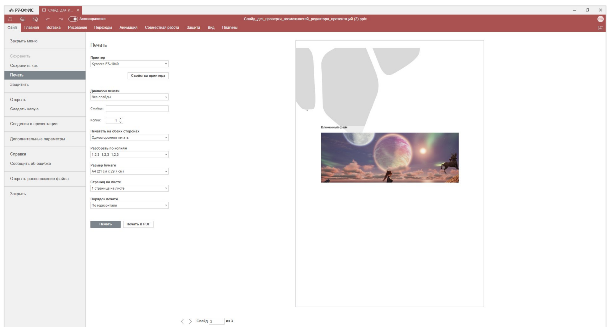
Рисунок 151 – Окно предпросмотра
