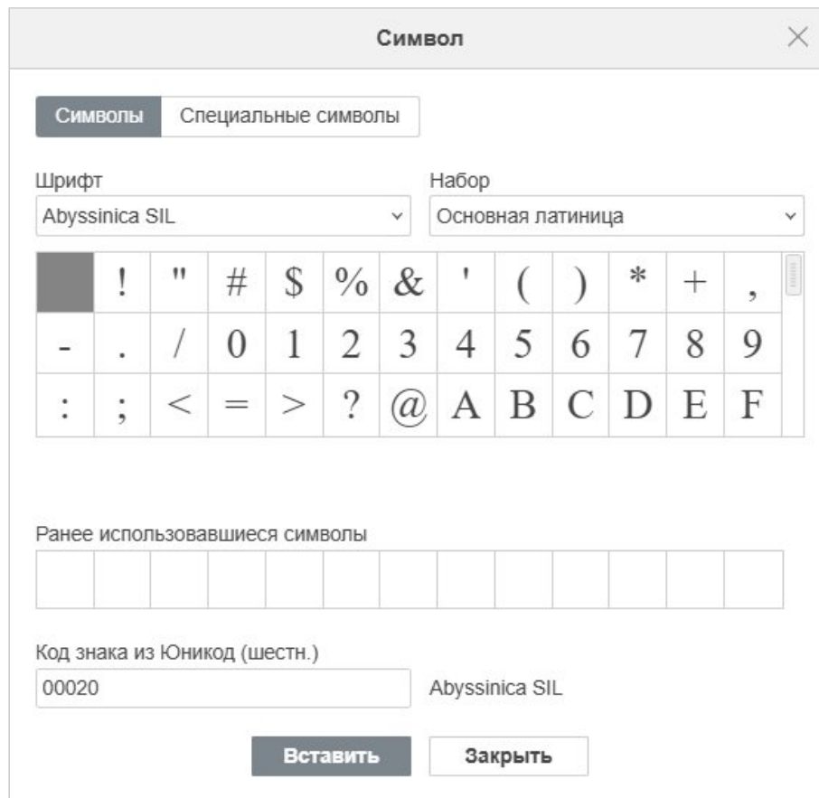
Рисунок 124 – Окно «Символ»
