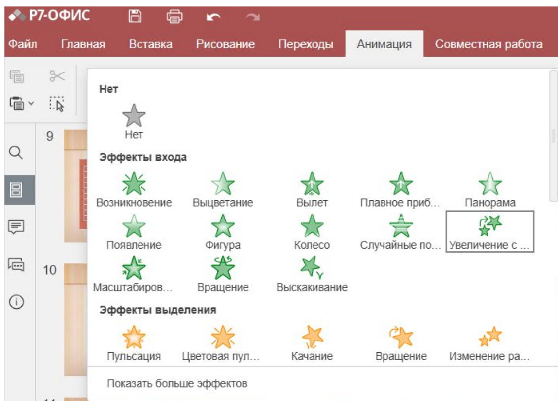
Рисунок 113 – Эффекты анимации
