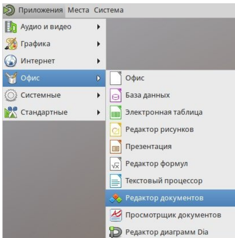
Рисунок 19 – Запуск ПО
