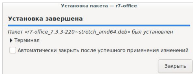
Рисунок 12 – Завершение установки
