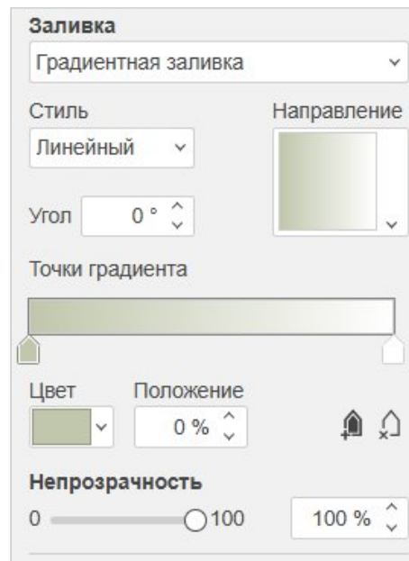
Рисунок 130 – Градиентная заливка
