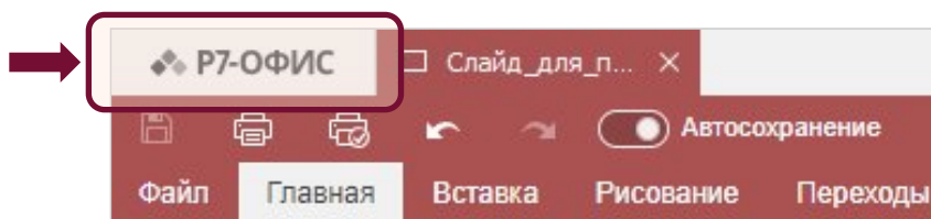
Рисунок 23 – Логотип «Р7-ОФИС»
