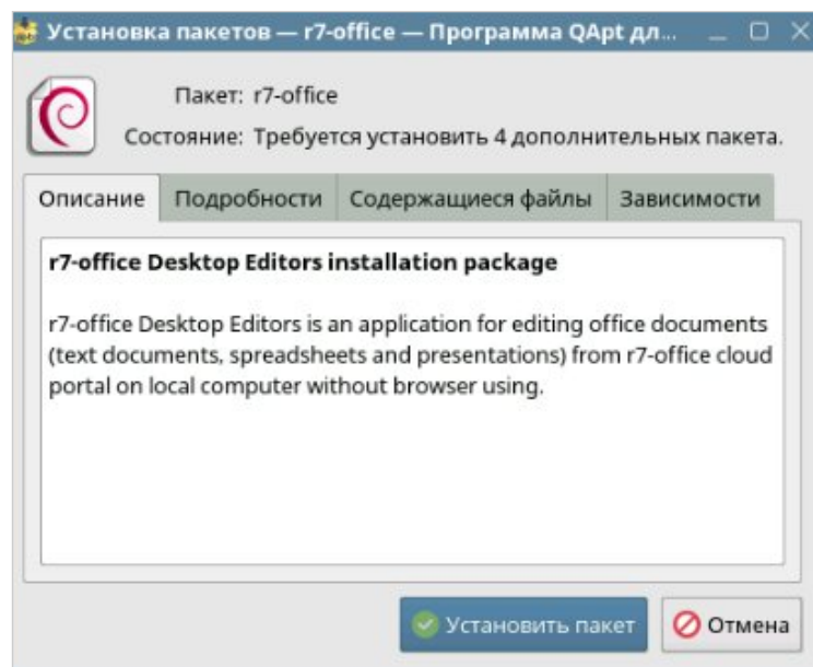
Рисунок 6 – Окно установки
