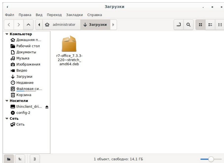
Рисунок 9 – Запуск дистрибутива
