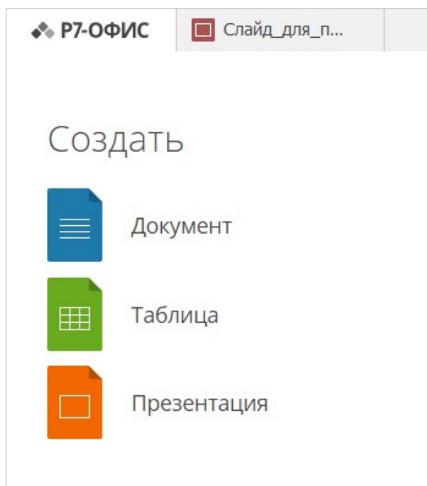
Рисунок 37 – Раздел «Создать»
