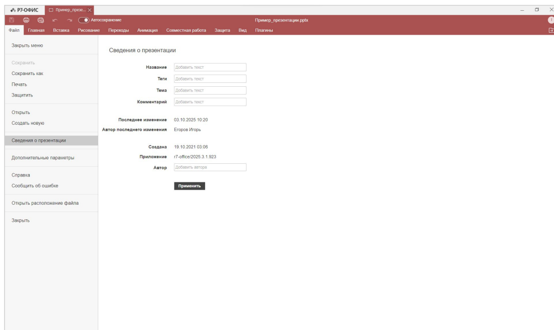
Рисунок 26 – Вкладка «Файл»
