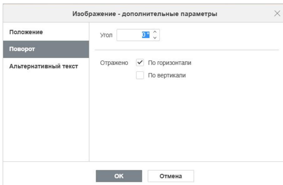
Рисунок 83 – Вкладка «Поворот»
