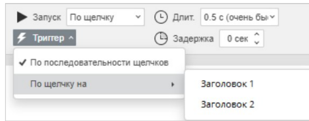
Рисунок 119 – Опции триггера
