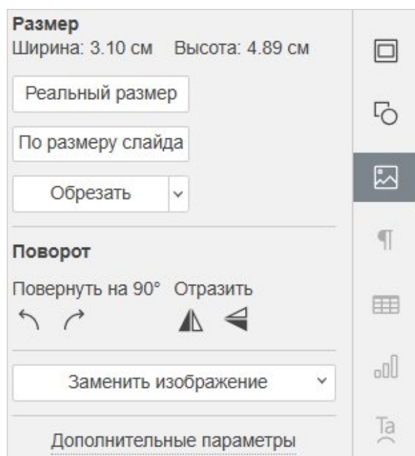
Рисунок 80 – Параметры изображения
