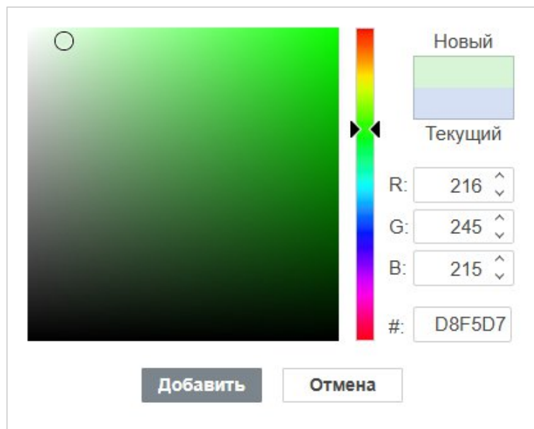
Рисунок 129 – Пользовательский цвет
