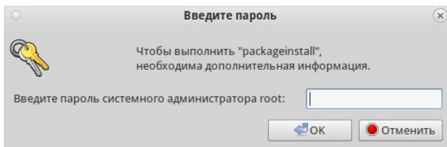
Рисунок 16 – Ввод пароля
