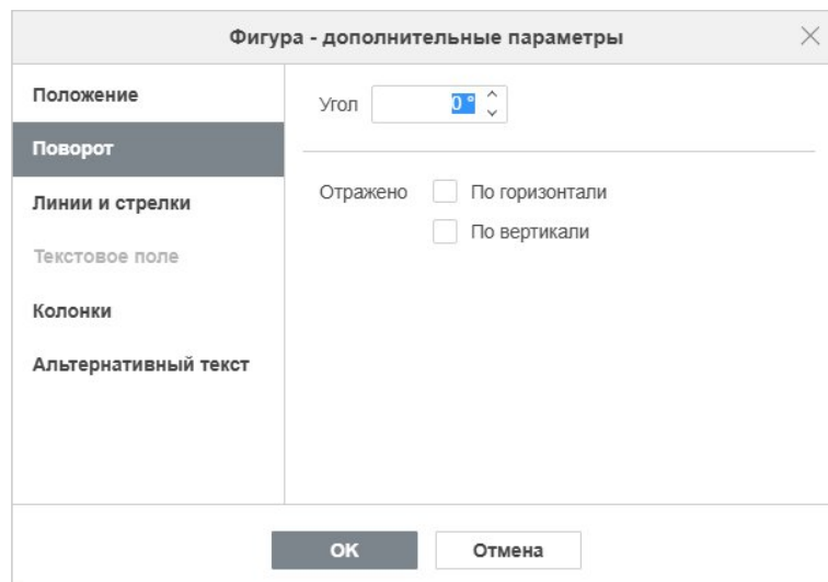
Рисунок 71 – Вкладка «Поворот»
