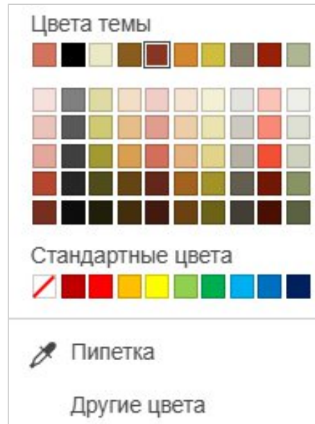
Рисунок 128 – Выбор цвета
