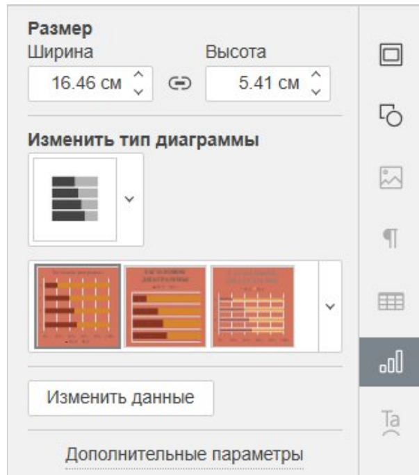
Рисунок 99 – Параметры диаграммы
