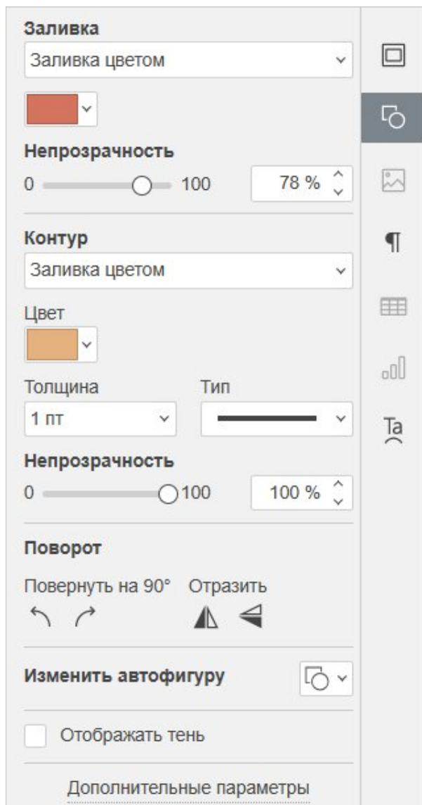
Рисунок 69 – Параметры фигуры
