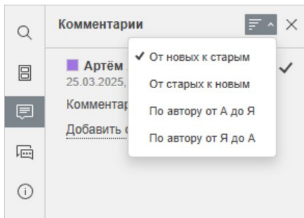
Рисунок 149 – Сортировка комментариев
