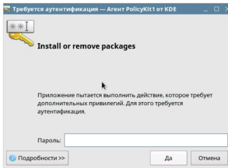
Рисунок 7 – Ввод пароля
