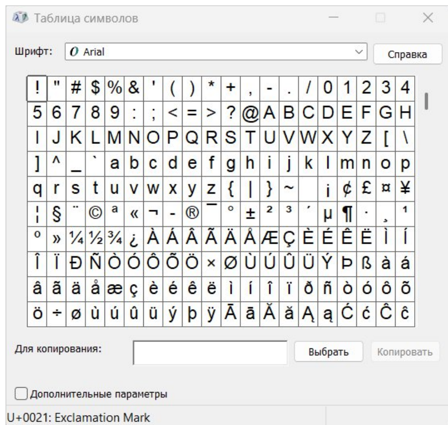
Рисунок 126 – Таблица символов
