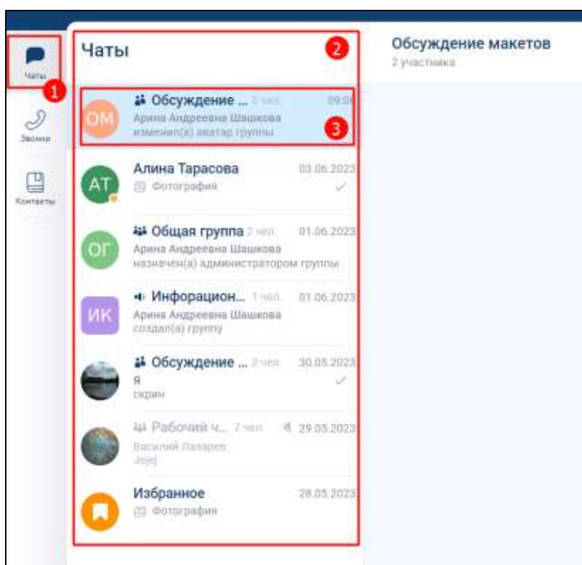
Рисунок 173 – Раздел «Чаты»
