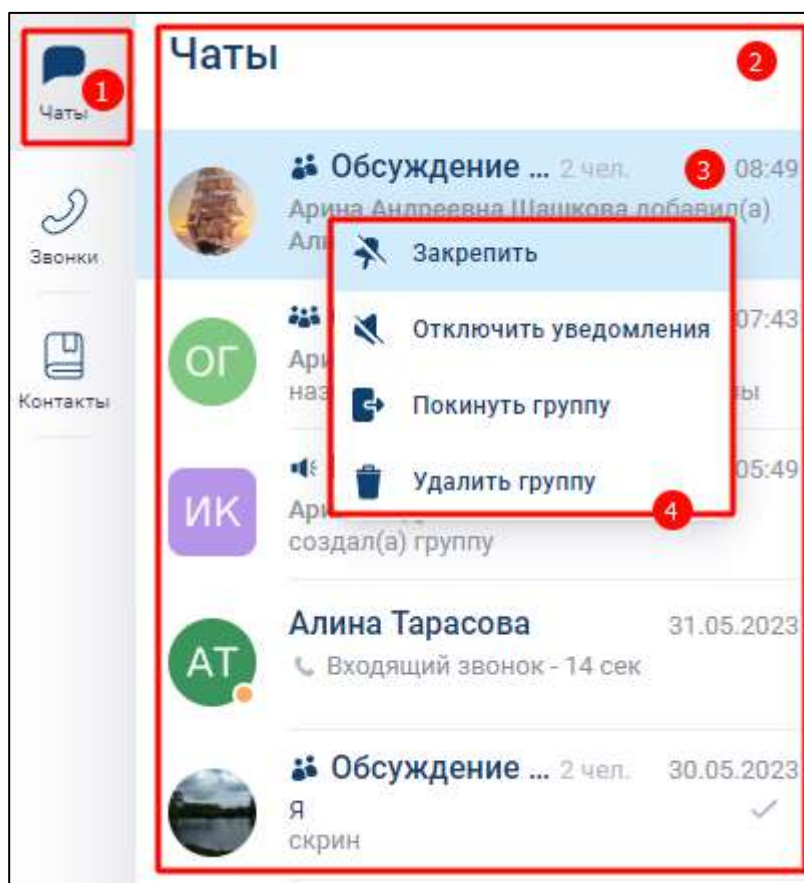
Рисунок 146- Раздел «Чаты»
