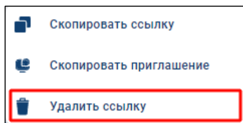
Рисунок 197 – Контекстное меню
