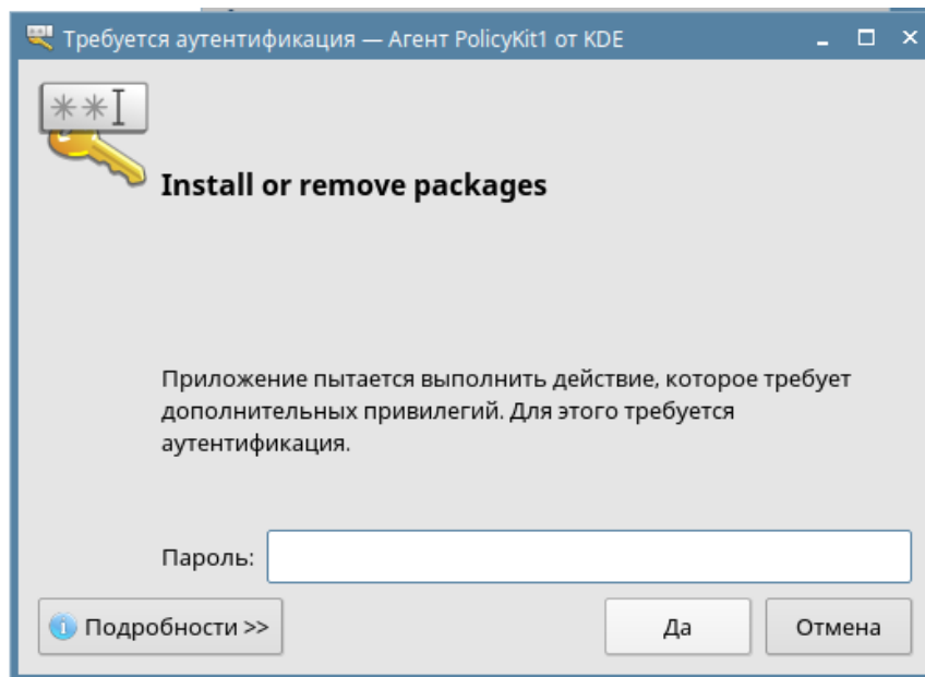
Рисунок 14 - Окно аутентификации
