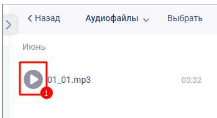
Рисунок 285 – Окно «Аудиофайлы»
