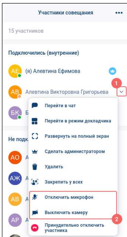
Рисунок 348 – Контекстное меню
