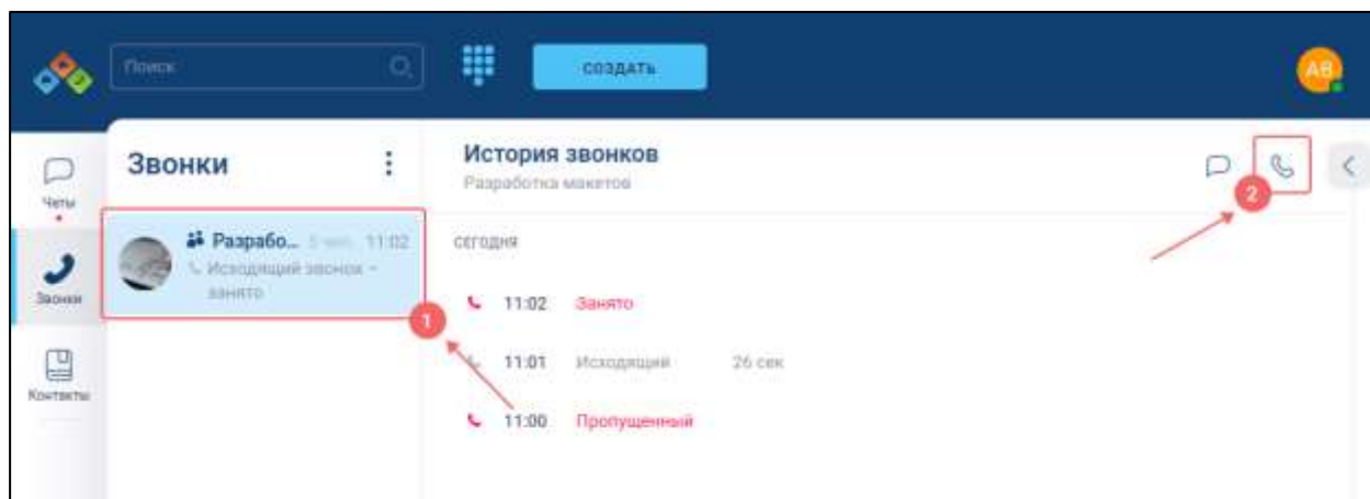
Рисунок 292 – Раздел «Звонки»
