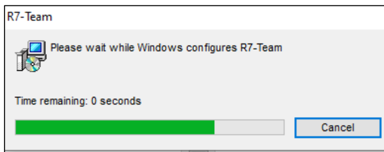
Рисунок 4 - Процесс установки
