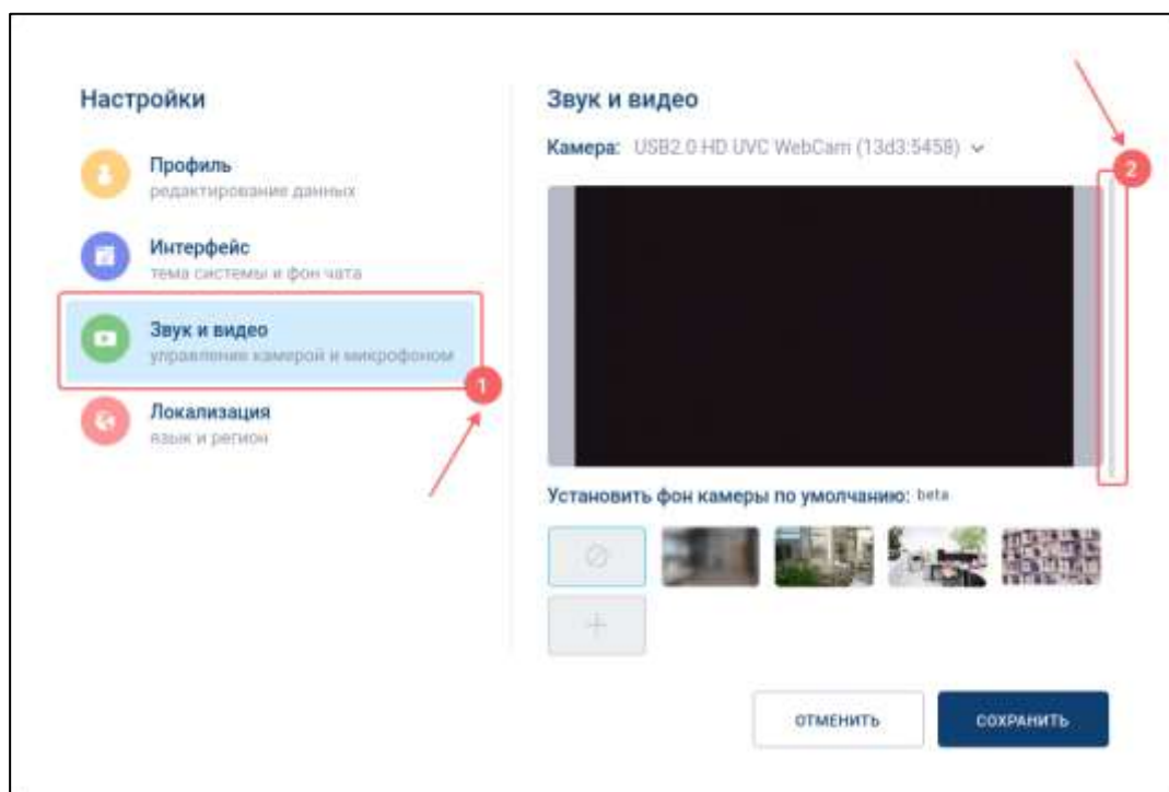
Рисунок 316 - Окно «Настройки»
