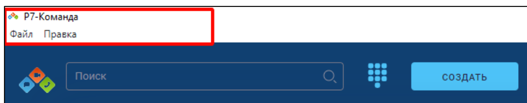
Рисунок 20 - Системное меню
