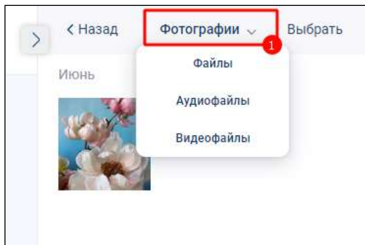
Рисунок 288 – Окно «Фотографии»
