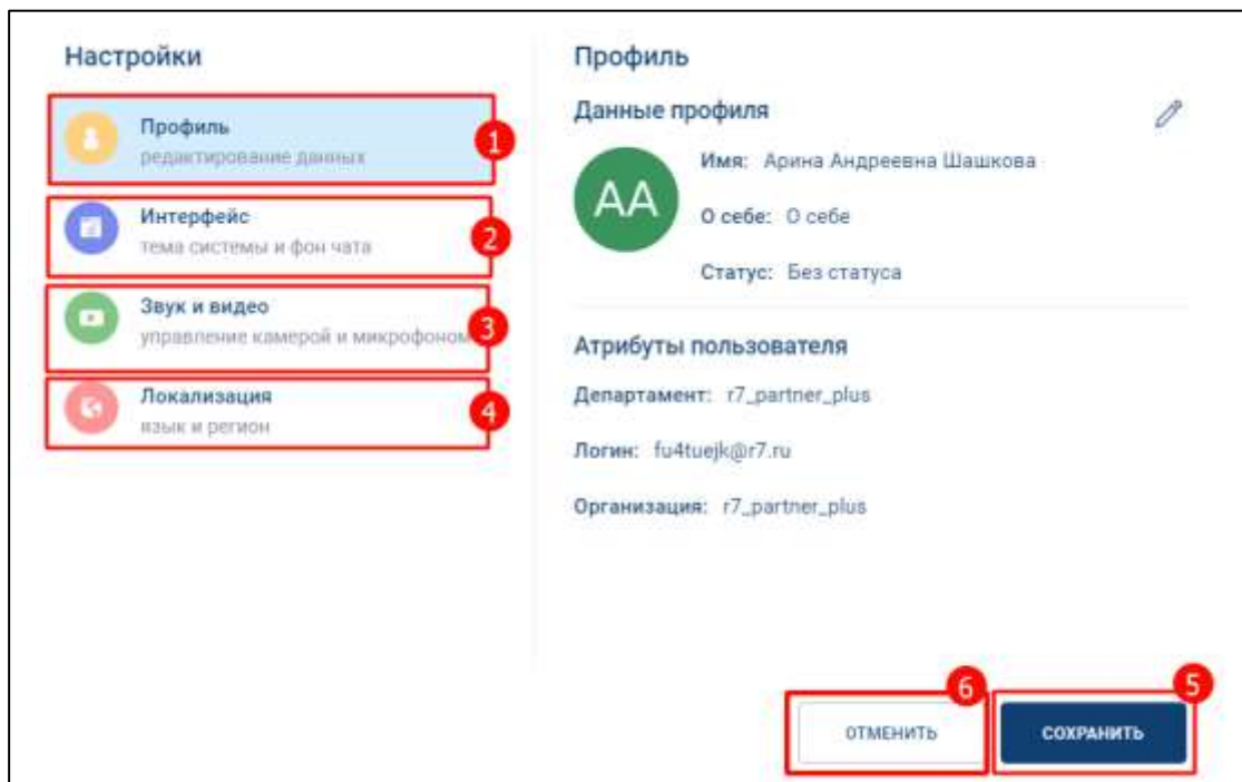
Рисунок 379 - Окно «Настройки»
