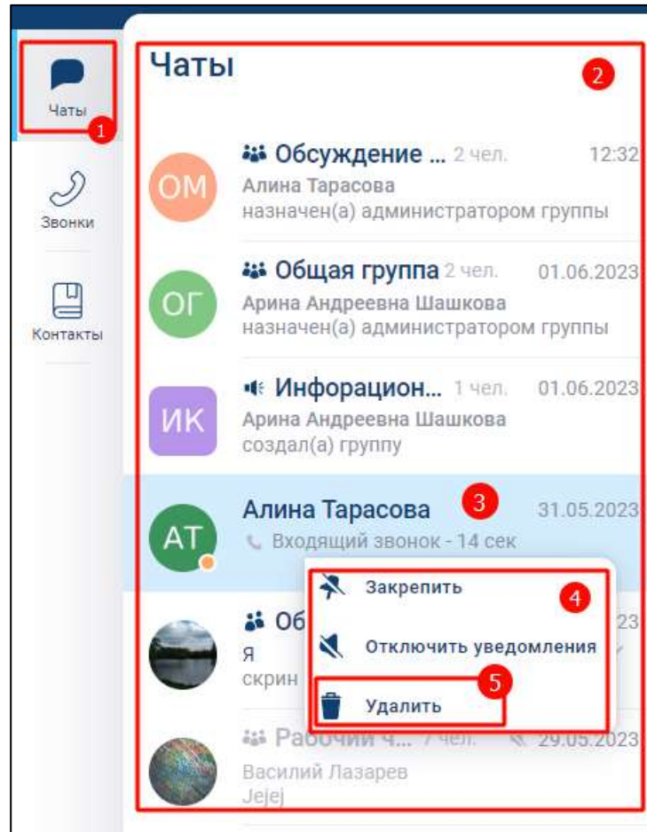
Рисунок 205 –Раздел «Чаты»
