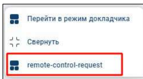
Рисунок 332 – Контекстное меню
