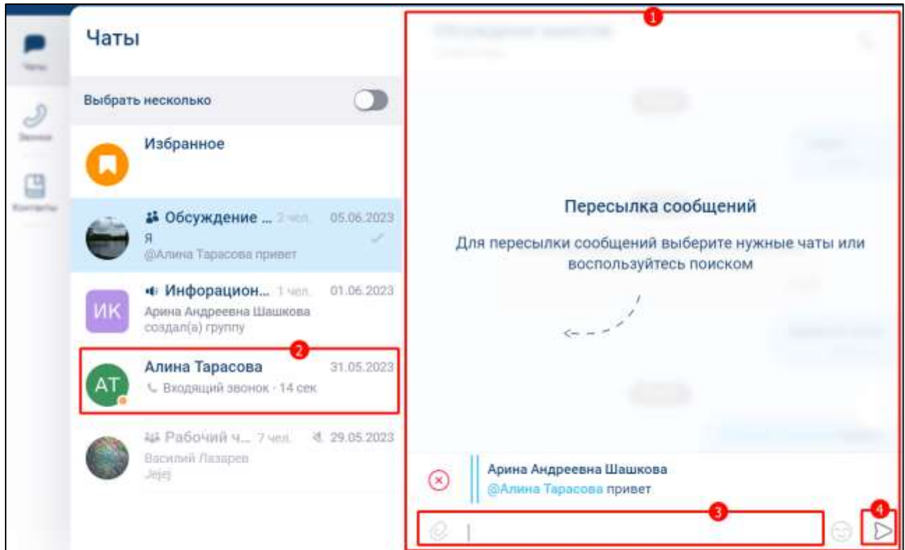
Рисунок 245 – Окно «Переслать»
