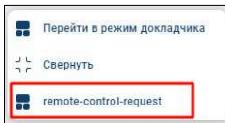
Рисунок 334 – Контекстное меню
