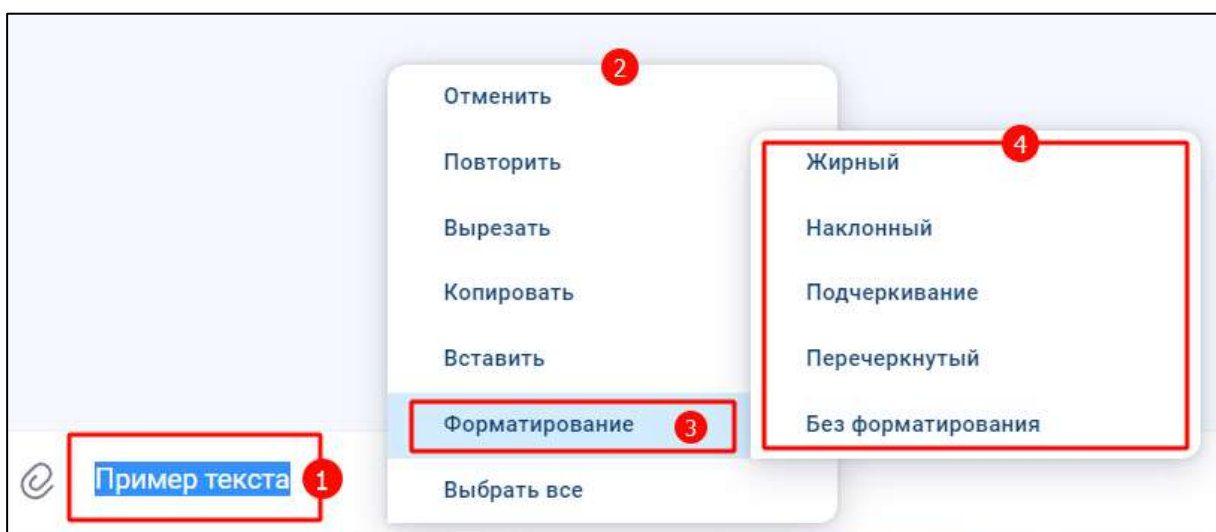
Рисунок 235 - Форматирование текста
