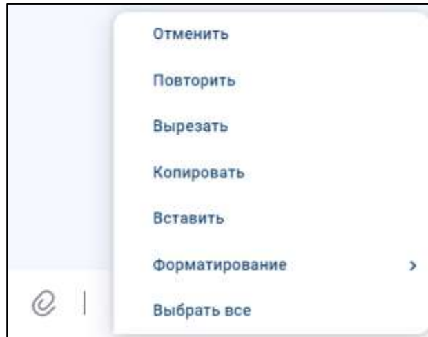
Рисунок 234 - Контекстное меню
