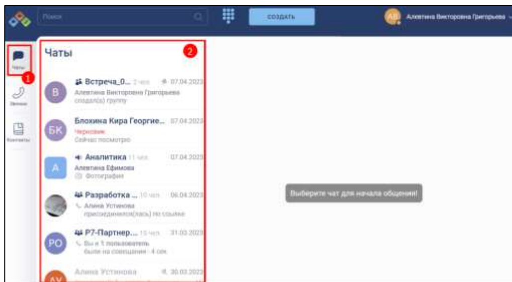
Рисунок 38 – Раздел «Чаты»
