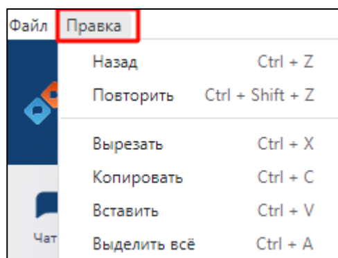
Рисунок 23 – Раздел «Правка»
