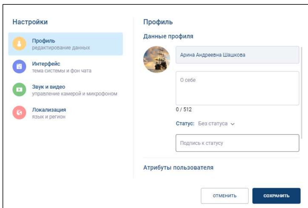
Рисунок 383 - Измененный аватар
