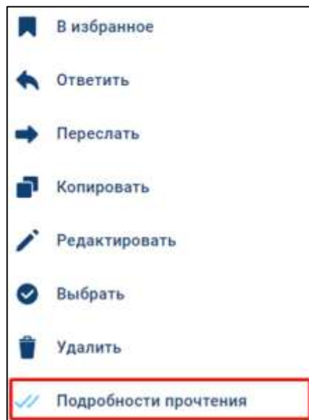
Рисунок 254 – Контекстное меню
