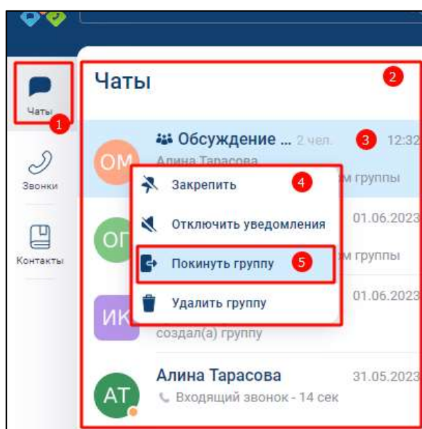
Рисунок 212 – Раздел «Чаты»
