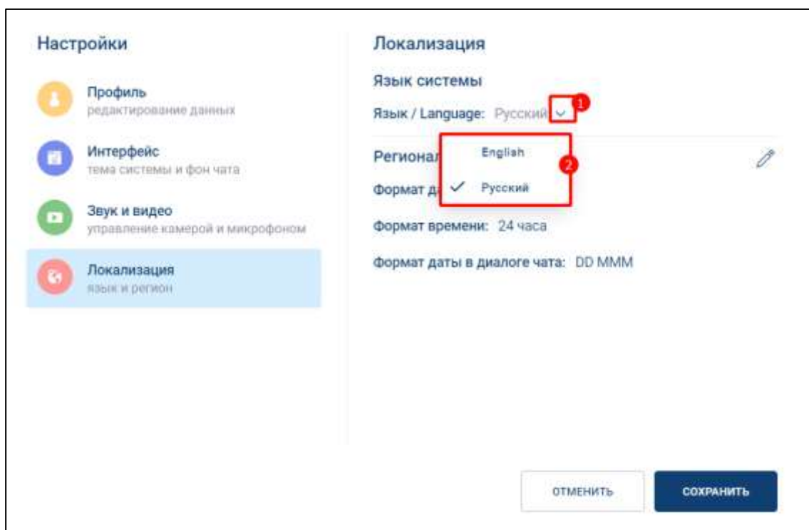
Рисунок 389 - Изменение языка
