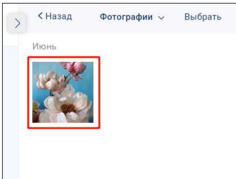
Рисунок 278 – Окно «Фотографии»
