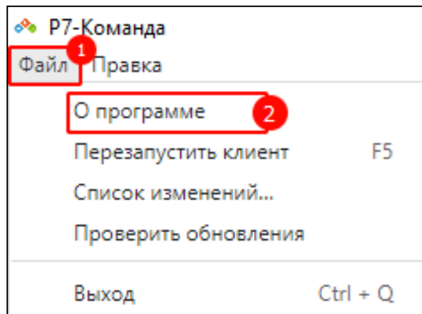
Рисунок 403 – Раздел «Файл»
