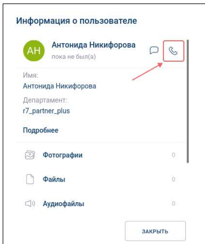
Рисунок 294 – Начало звонка через окно информации о пользователе
