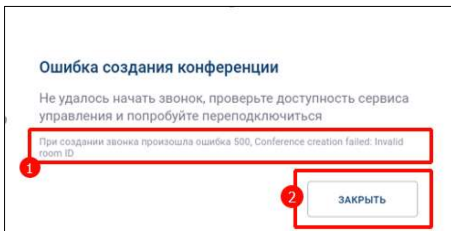
Рисунок 362 - Подробное описание ошибки
