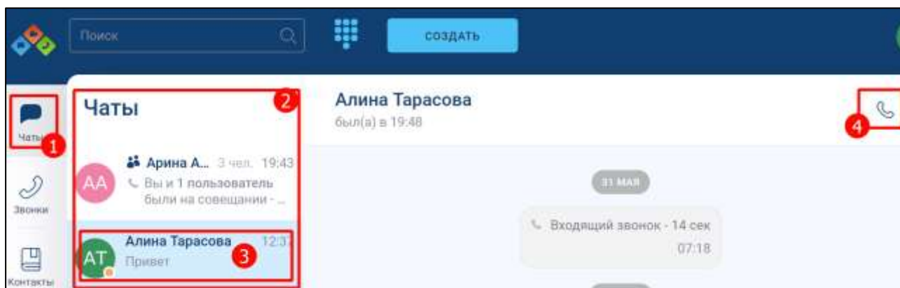
Рисунок 113 –Раздел «Чаты»
