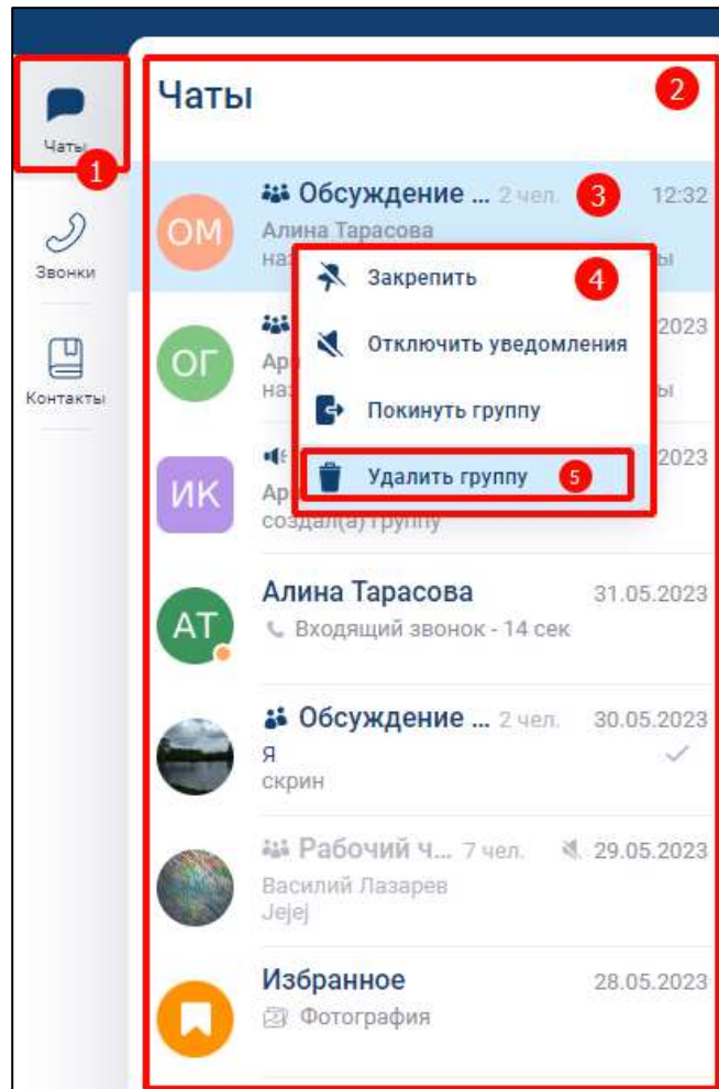
Рисунок 208 – Раздел «Чаты»
