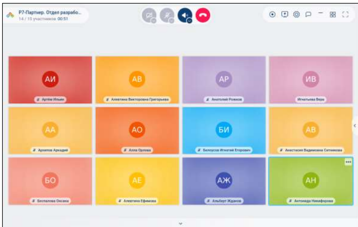
Рисунок 338 - Режим «Мозаика»
