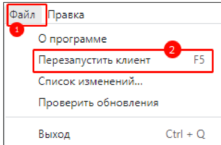
Рисунок 405 - Раздел «Файл»
