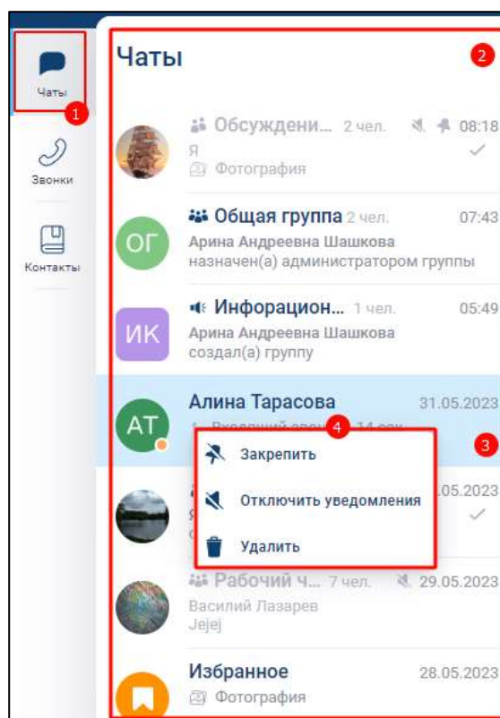
Рисунок 143 –Раздел «Чаты»
