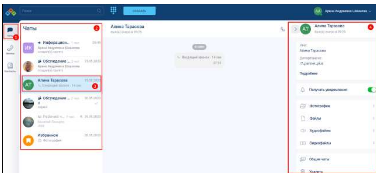
Рисунок 144 - Раздел «Чаты»
