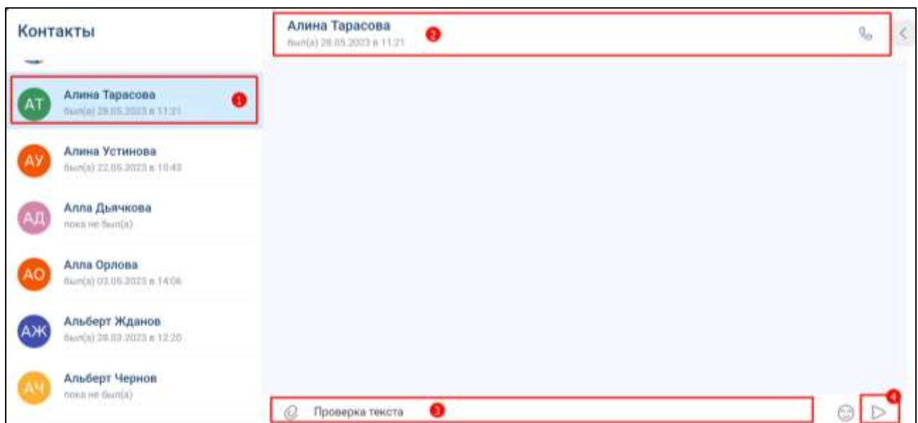
Рисунок 108 – Раздел «Контакты»
