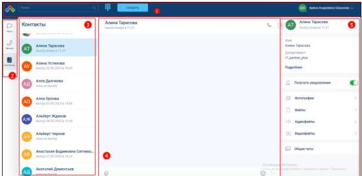
Рисунок 19 – Главная страница
