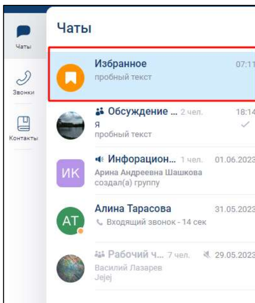
Рисунок 219 – Чат «Избранное»
