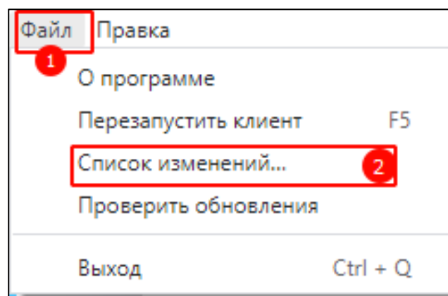
Рисунок 406 – Раздел «Файл»
