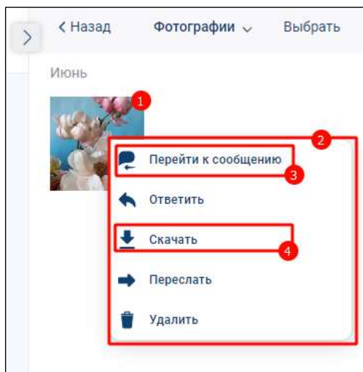
Рисунок 289- Контекстное меню
