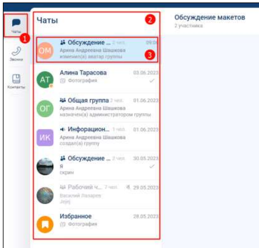
Рисунок 168 – Раздел «Чаты»
