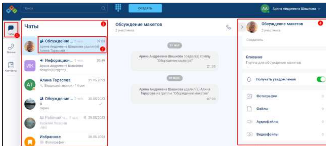
Рисунок 140 – Раздел «Чаты»
