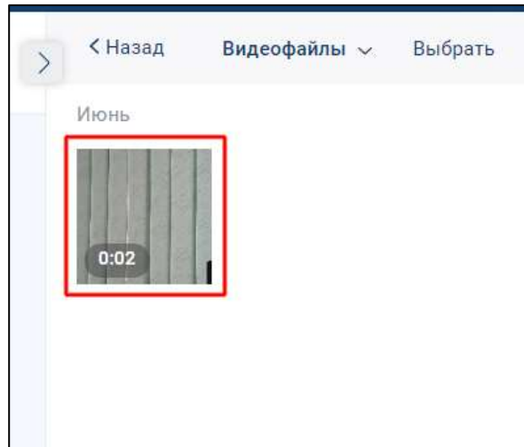
Рисунок 281 – Окно «Вложения»
