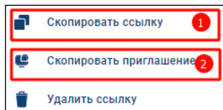
Рисунок 196 – Контекстное меню
