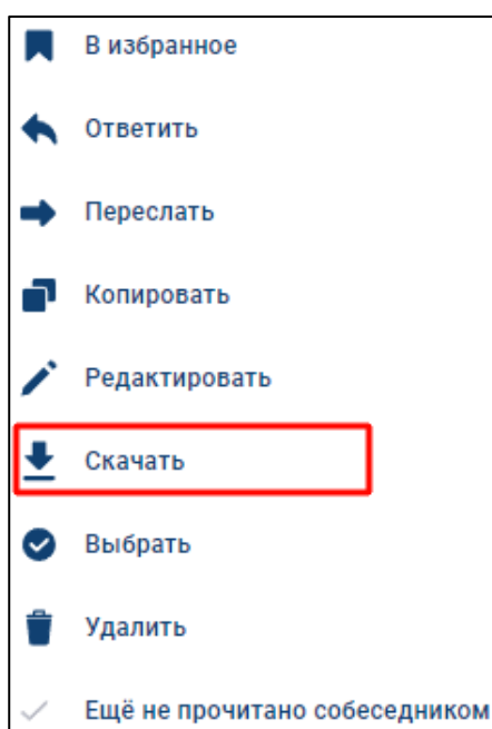
Рисунок 286 – Контекстное меню
