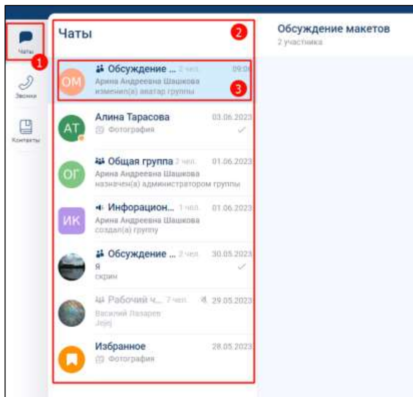
Рисунок 158 – Раздел «Чаты»
