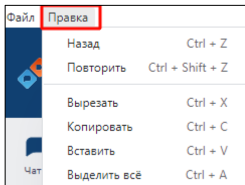
Рисунок 24 – Раздел «Правка»
