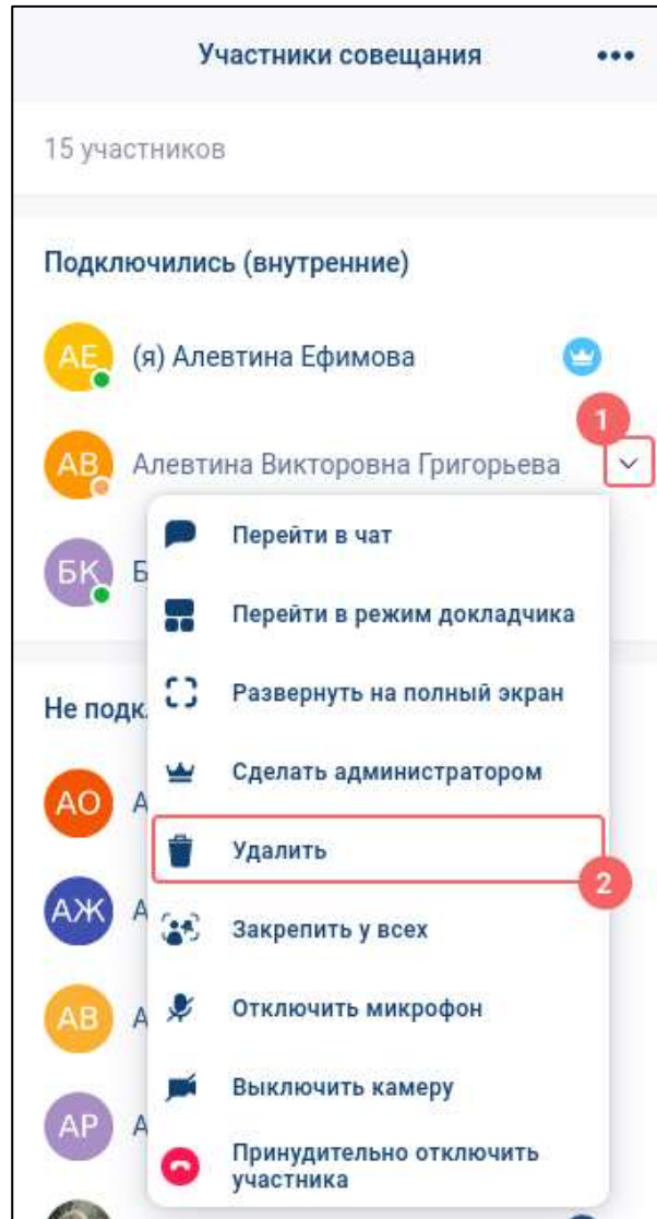
Рисунок 354 – Контекстное меню
