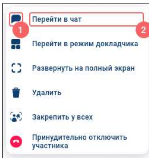
Рисунок 93 – Контекстное меню
