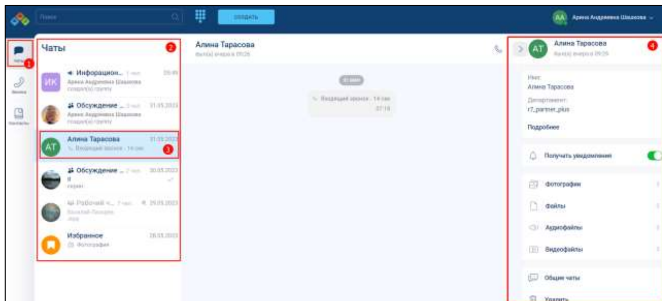
Рисунок 136 - Раздел «Чаты»
