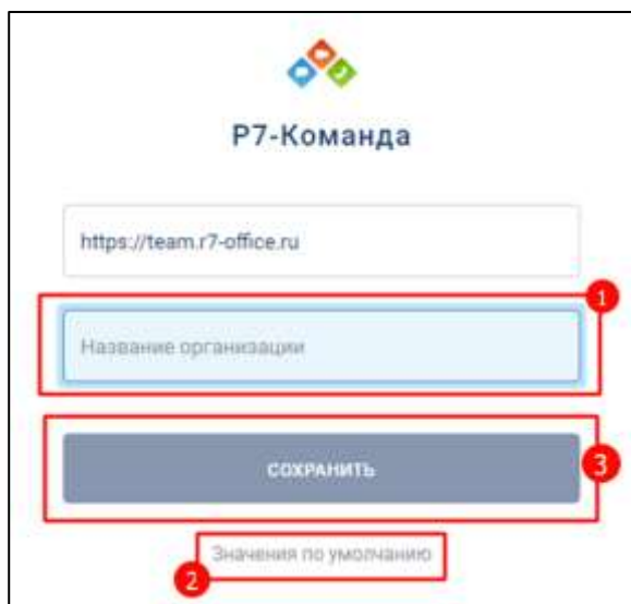
Рисунок 17 – Окно авторизации
