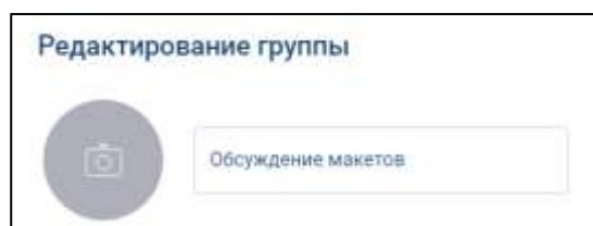
Рисунок 156 – Удаленный аватар
