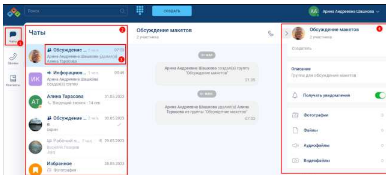
Рисунок 148 – Раздел «Чаты»
