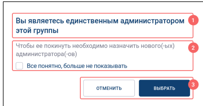
Рисунок 92 – Диалоговое окно
