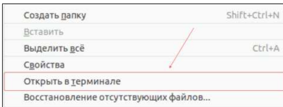
Рисунок 8 - Контекстное меню
