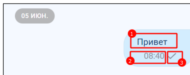
Рисунок 226 - Отправленное сообщение
