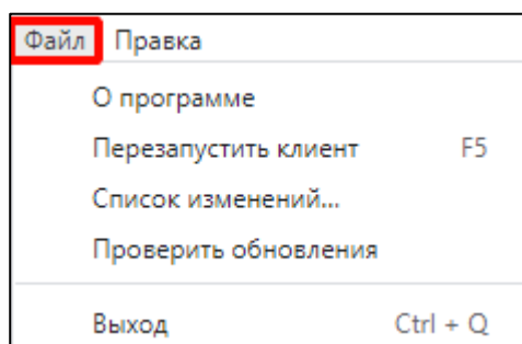
Рисунок 22 – Раздел «Файл»
