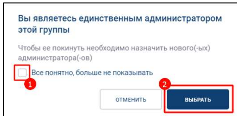
Рисунок 213 – Сообщение-предупреждение
