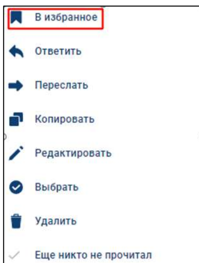
Рисунок 218- Контекстное меню
