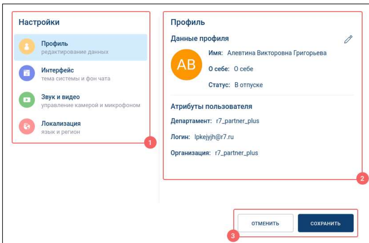
Рисунок 32 – Окно «Настройки»
