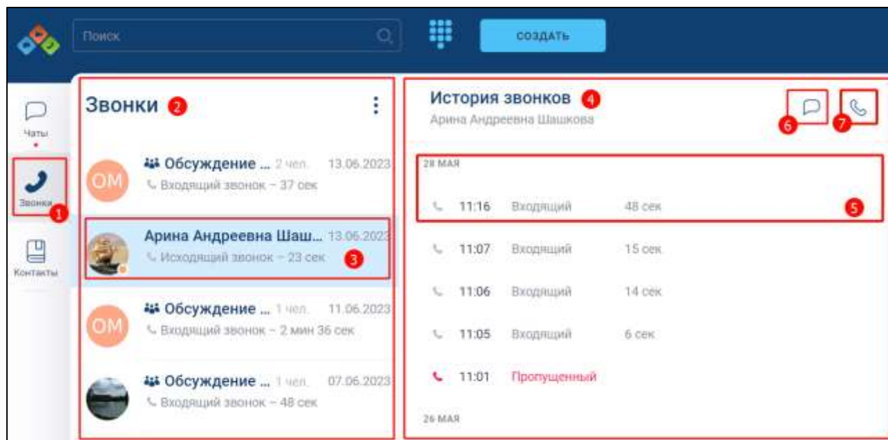
Рисунок 367 - Раздел «Звонки»
