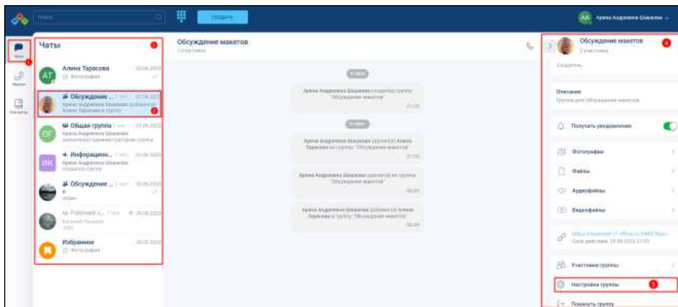
Рисунок 150 – Раздел «Чаты»
