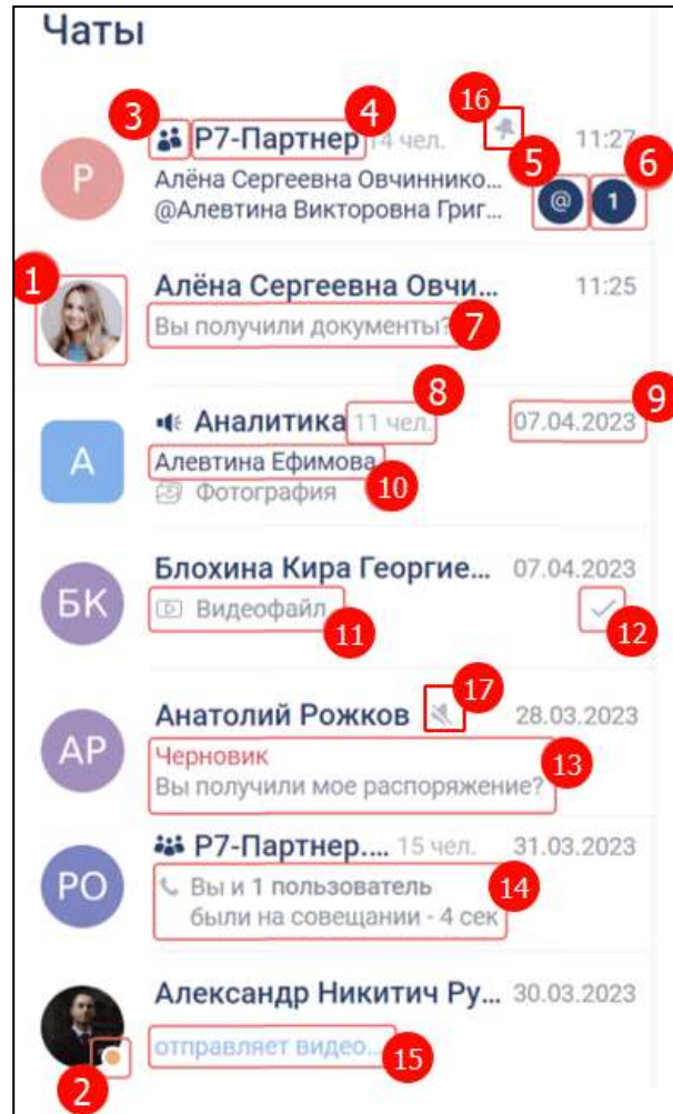
Рисунок 39 – Список чатов
