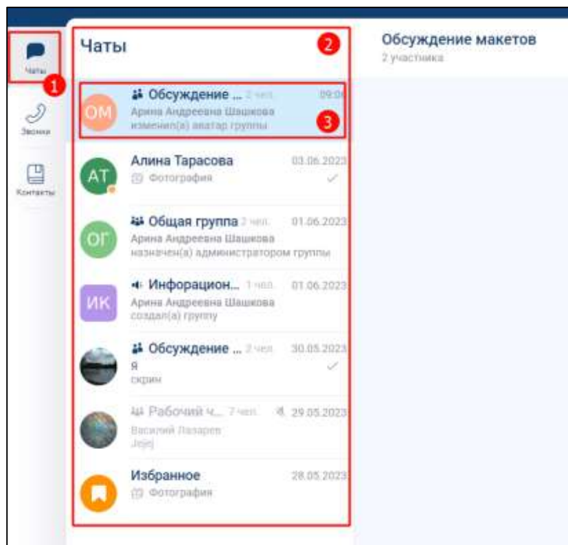
Рисунок 187 – Раздел «Чаты»
