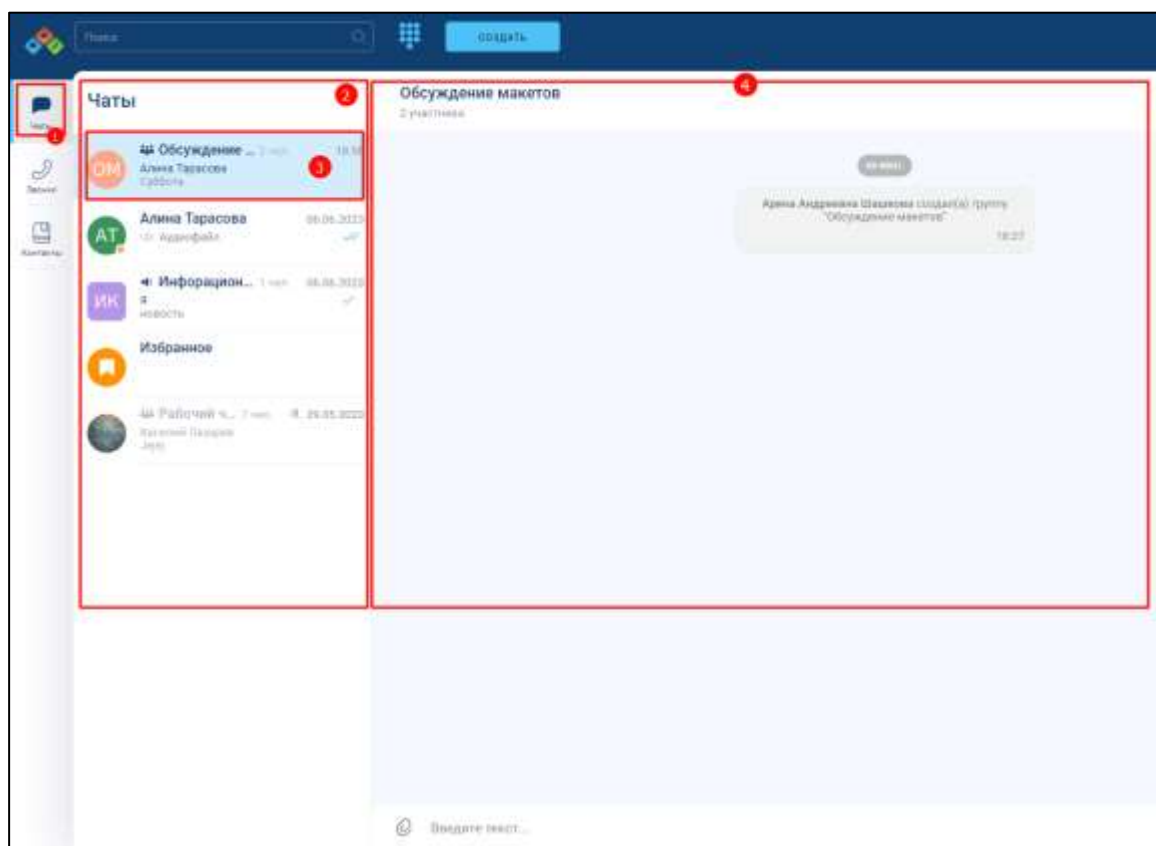
Рисунок 271 – Раздел «Чаты»
