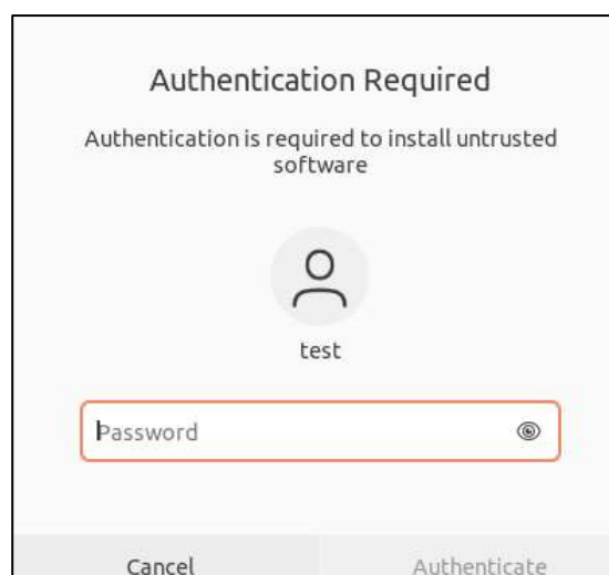
Рисунок 12 - Окно аутентификации
