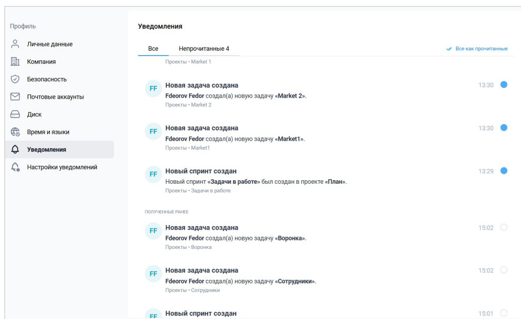
Рисунок 186 – Раздел «Уведомления»
