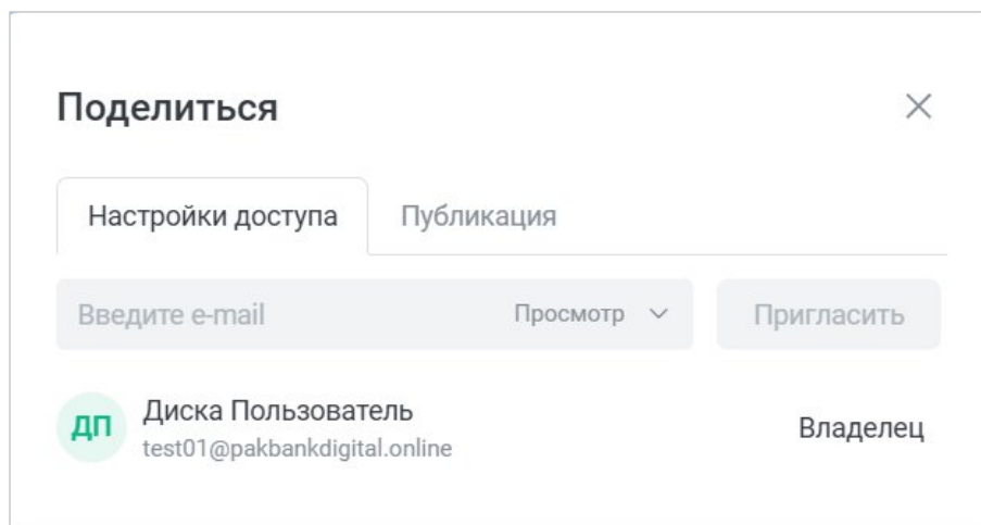
Рисунок 143 – Функция «Поделиться»
