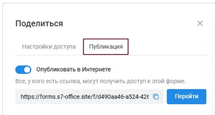
Рисунок 166 – Вкладка «Публикация»
