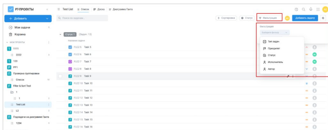
Рисунок 98 – Фильтрация задач
