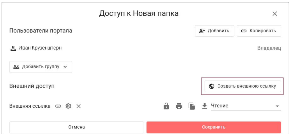
Рисунок 23 – Окно «Доступ»
