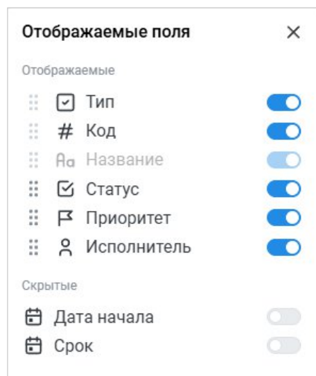
Рисунок 100 – Настройка полей
