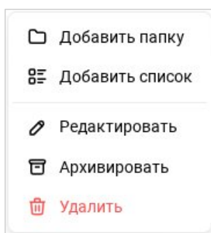
Рисунок 107 – Выпадающий список
