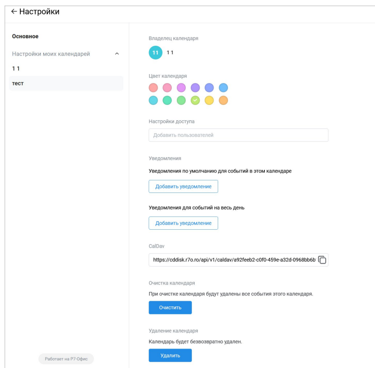
Рисунок 45 – Настройки календарей
