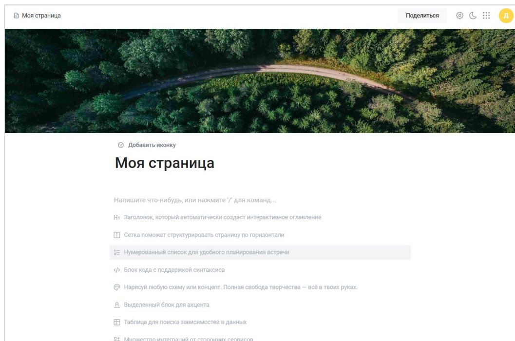
Рисунок 134 – Рабочая область
