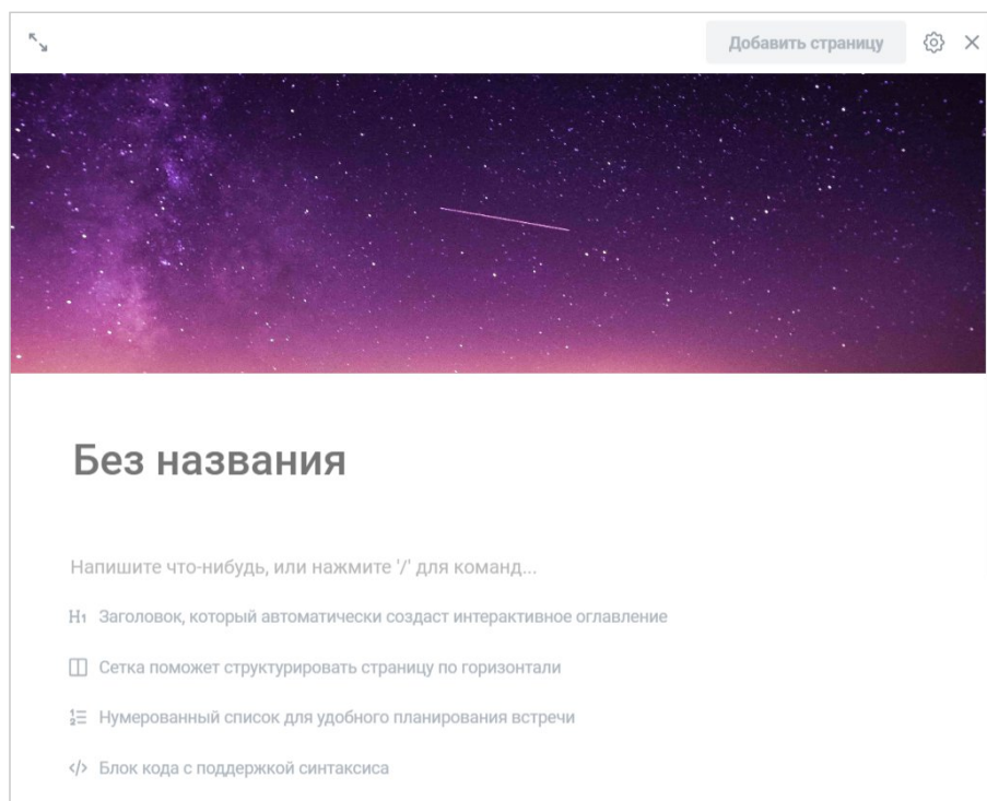
Рисунок 131 – Создание страницы
