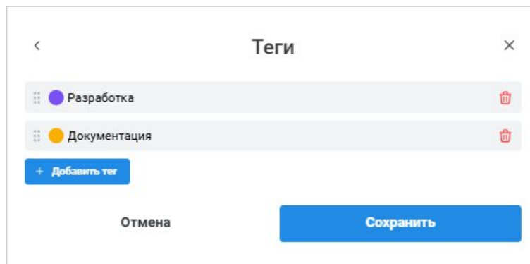
Рисунок 105 – Окно «Теги»
