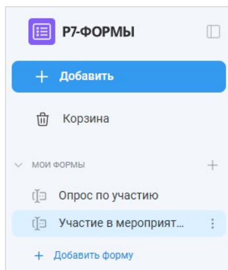
Рисунок 148 – Боковая панель
