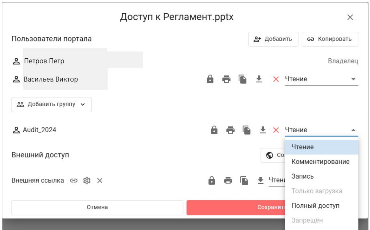
Рисунок 21 – Предоставление доступа
