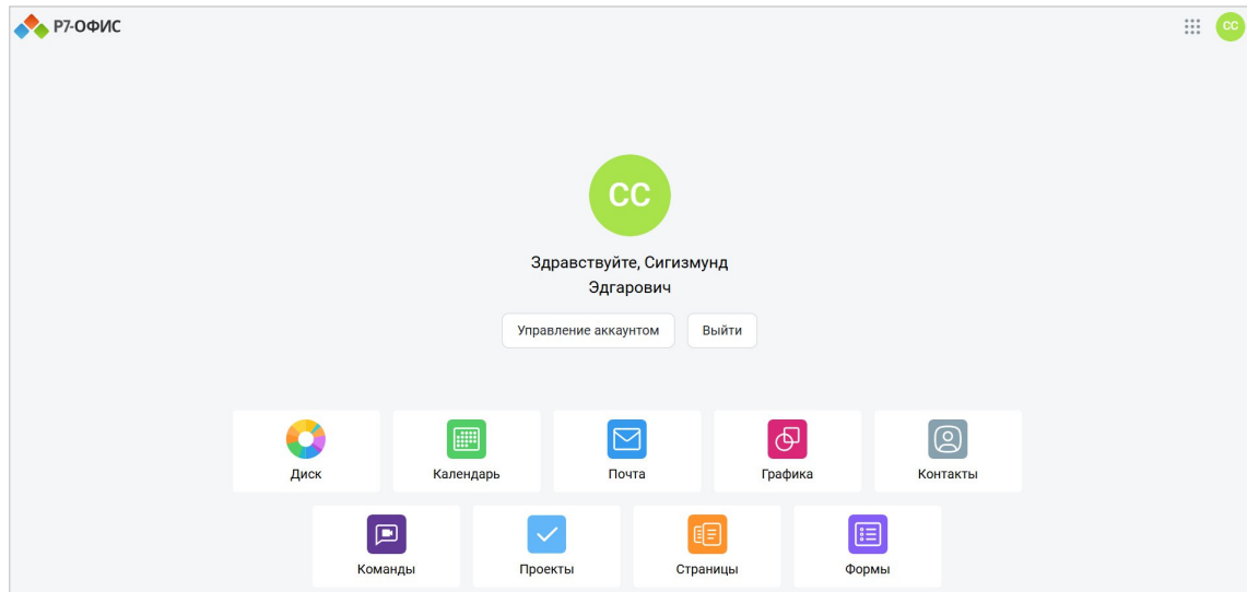
Рисунок 2 – Главная страница
