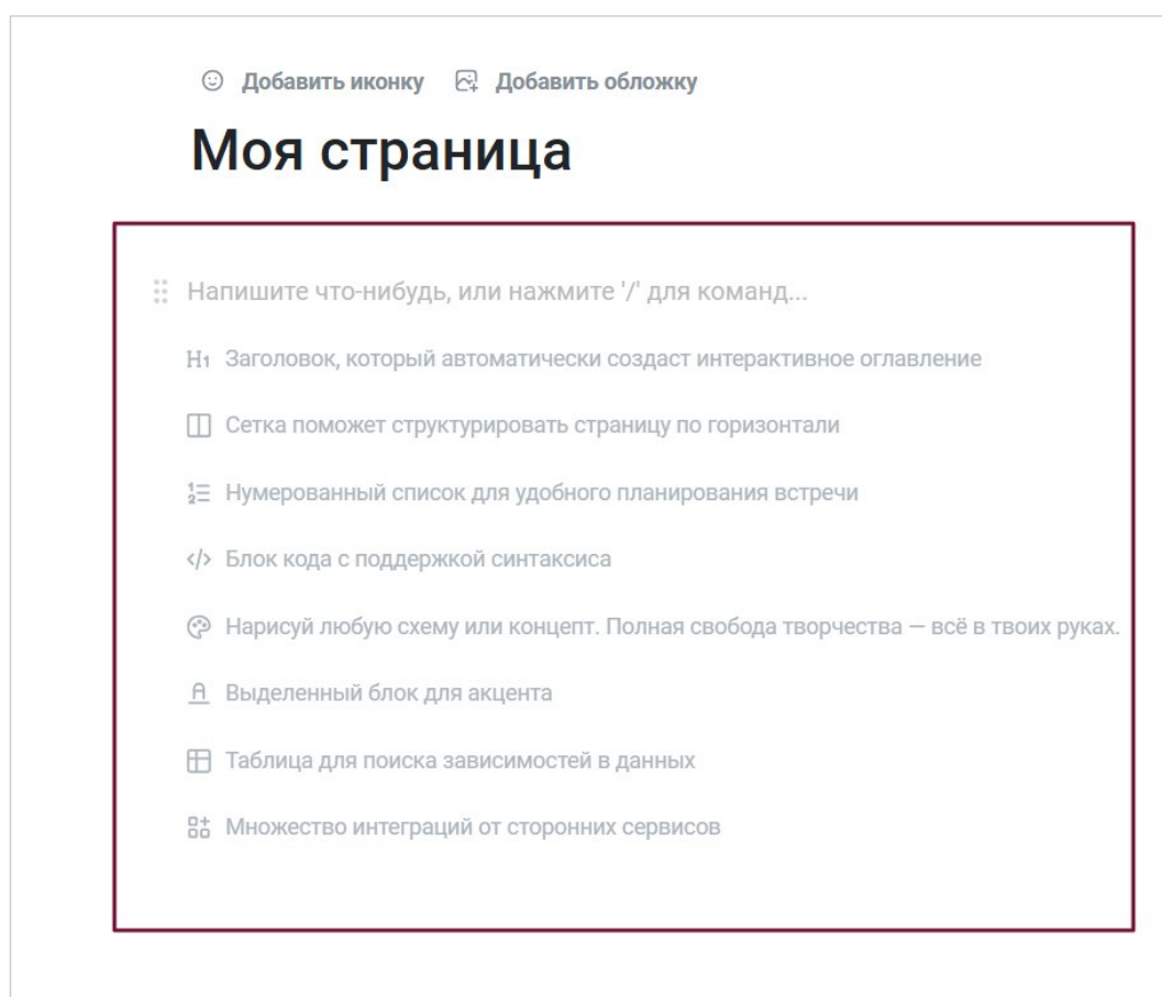
Рисунок 141 – Типы блоков
