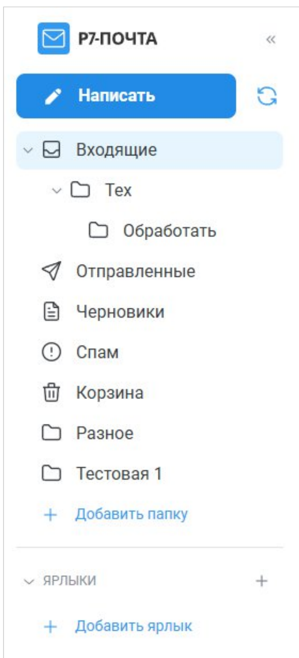
Рисунок 63 – Пользовательские папки
