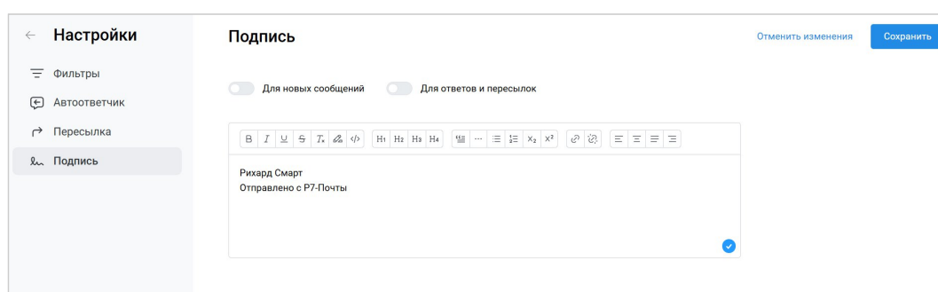
Рисунок 75 – Настройка подписи
