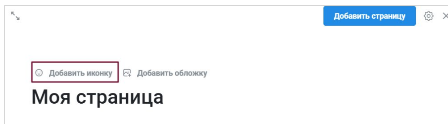
Рисунок 136 – Добавление иконки
