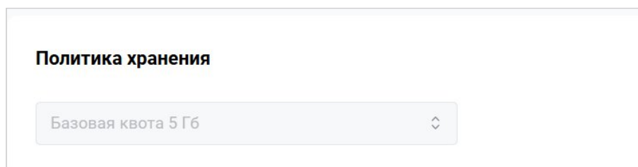
Рисунок 184 – Раздел «Диск»
