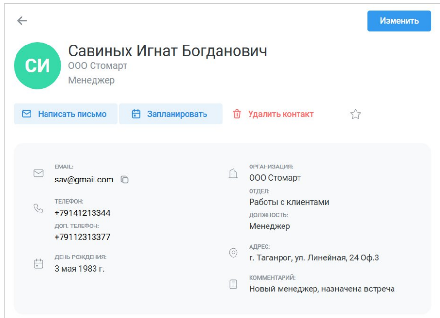
Рисунок 88 – Карточка контакта
