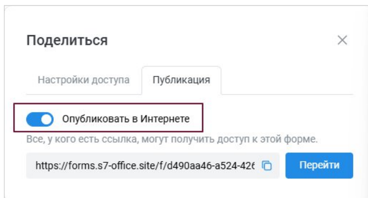
Рисунок 167 – Активация тумблера
