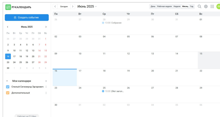
Рисунок 36 – Страница «Календарь»
