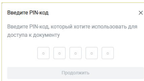
Рисунок 144 – Введение пин-кода
