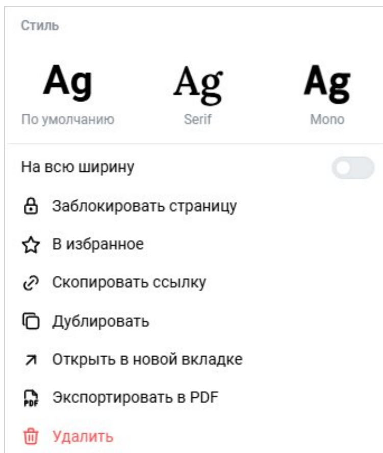
Рисунок 145 – Настройки страницы
