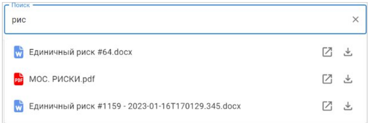
Рисунок 8 – Поиск
