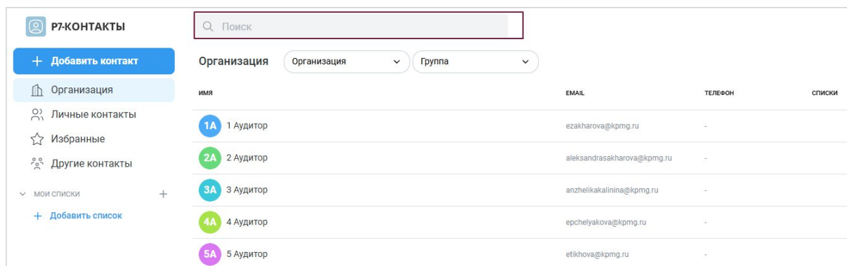
Рисунок 95 – Поле поиска
