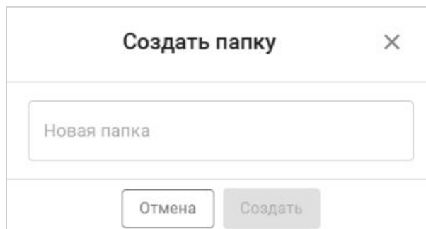
Рисунок 10 – Создание папки/документа
