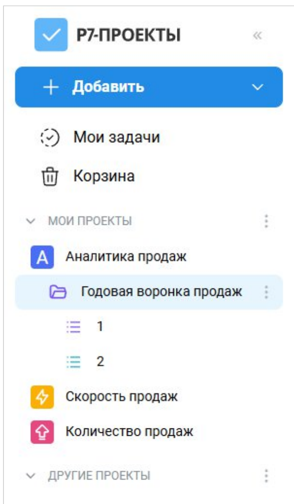
Рисунок 97 – Боковая панель
