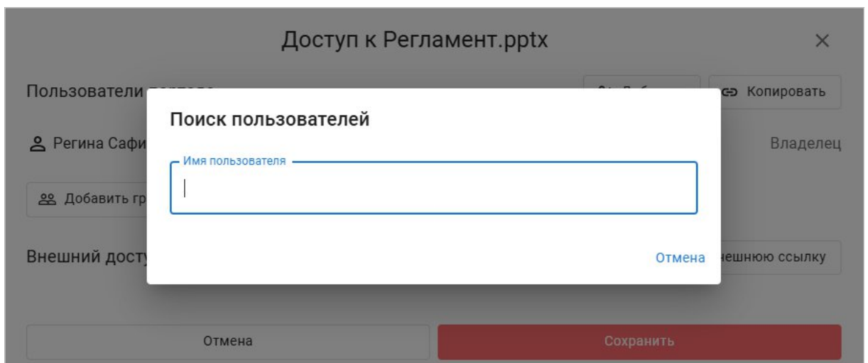
Рисунок 19 – Выбор пользователя
