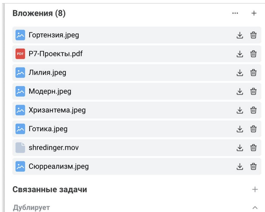
Рисунок 127 – Список вложений
