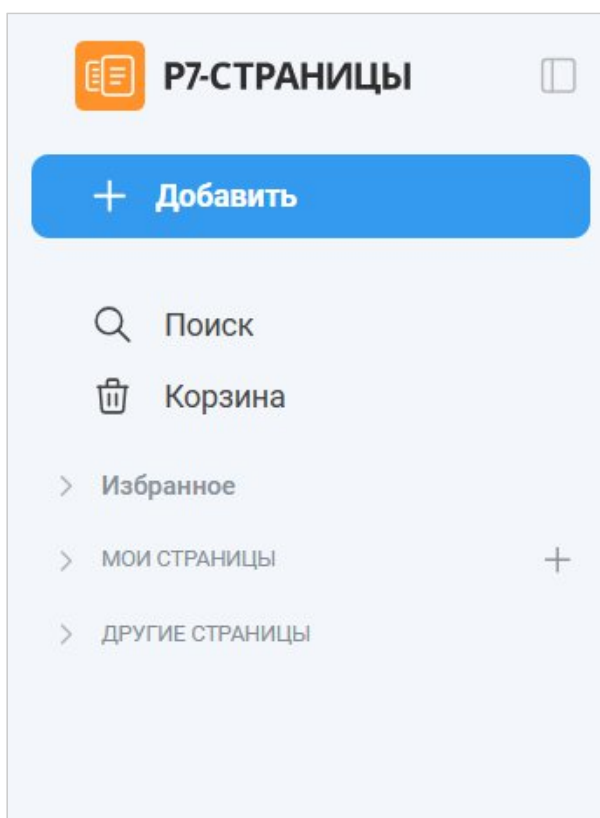
Рисунок 130 – Боковая панель
