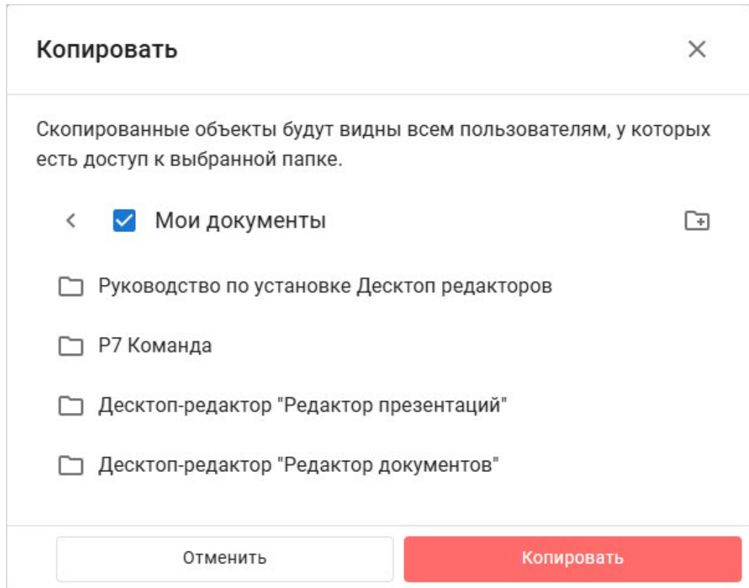
Рисунок 25 – Копирование
