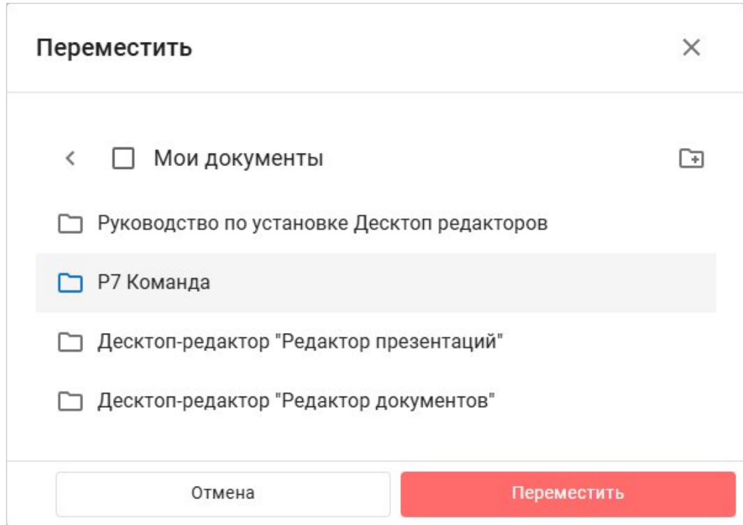
Рисунок 27 – Перемещение
