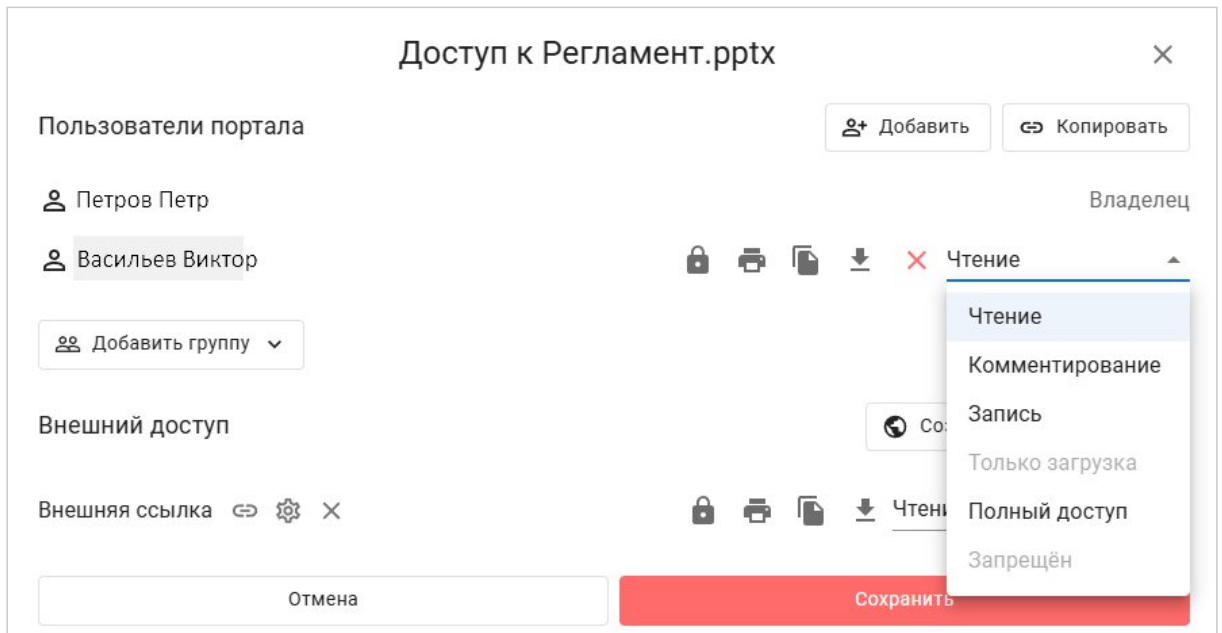
Рисунок 20 – Предоставление доступа
