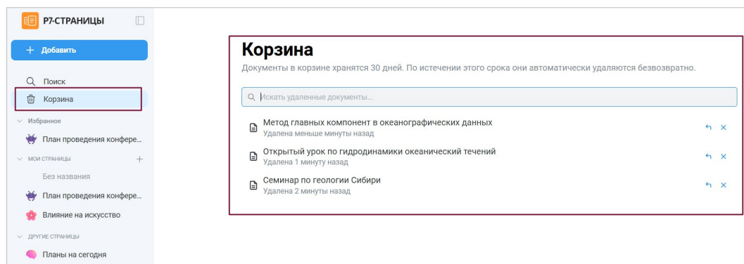
Рисунок 133 – Корзина
