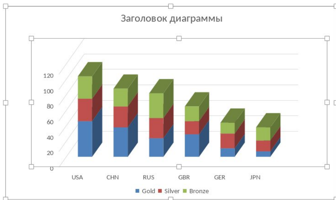
Рисунок 118 – 3D-диаграмма
