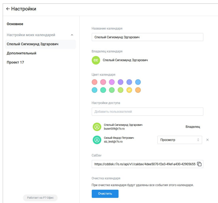
Рисунок 45 – Настройки календарей
