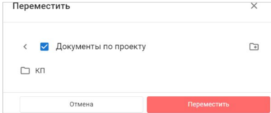
Рисунок 27 – Перемещение
