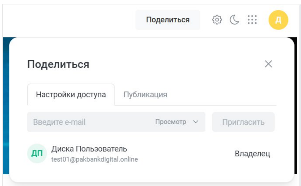
Рисунок 137 – Функция «Поделиться»
