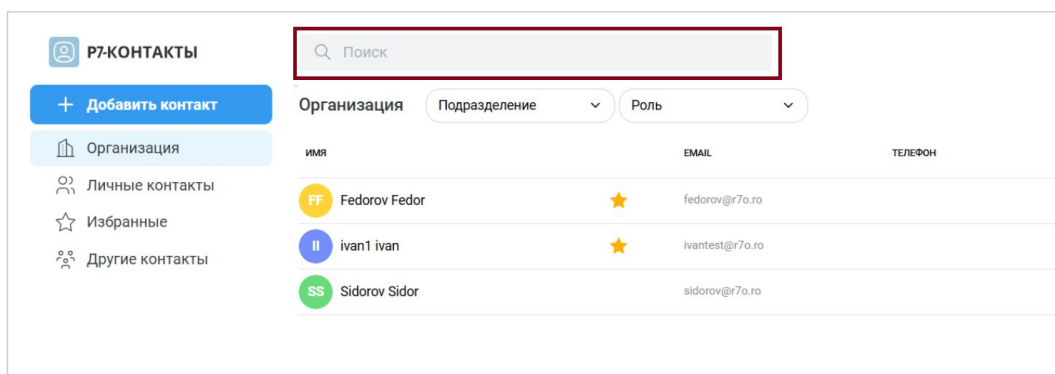
Рисунок 95 – Поле поиска
