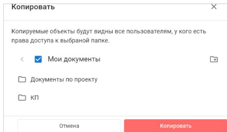
Рисунок 25 – Копирование
