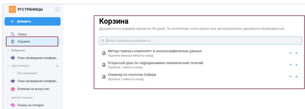
Рисунок 127 – Корзина
