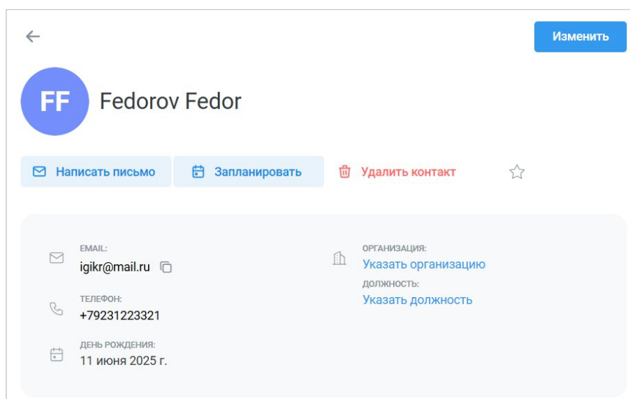
Рисунок 94 – Карточка контакта
