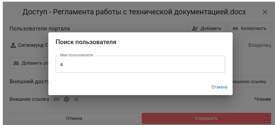
Рисунок 19 – Выбор пользователя
