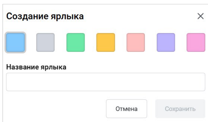
Рисунок 64 – Создание ярлыка
