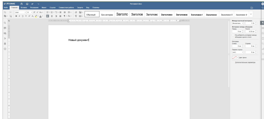
Рисунок 17 – Редактор
