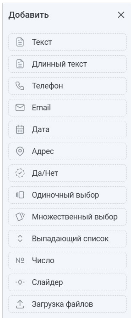
Рисунок 154 — Типы полей
