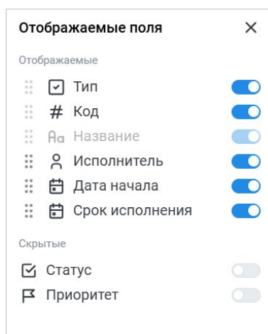
Рисунок 98 – Настройка полей
