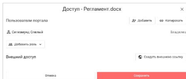
Рисунок 18 – Управление доступом
