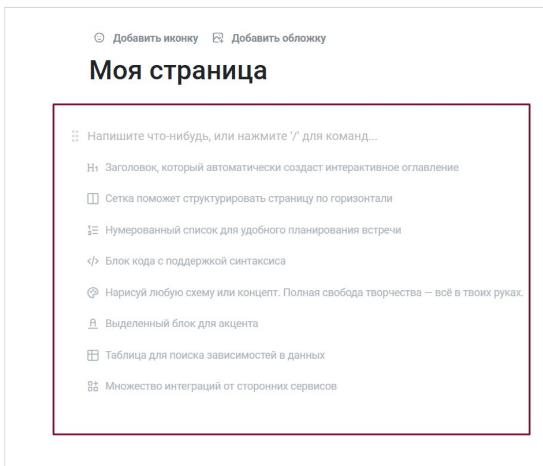
Рисунок 135 – Типы блоков
