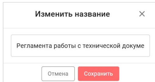
Рисунок 14 – Переименование документа
