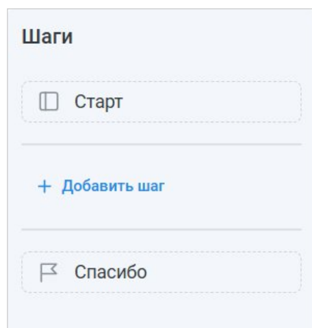
Рисунок 153 – Стартовый шаг
