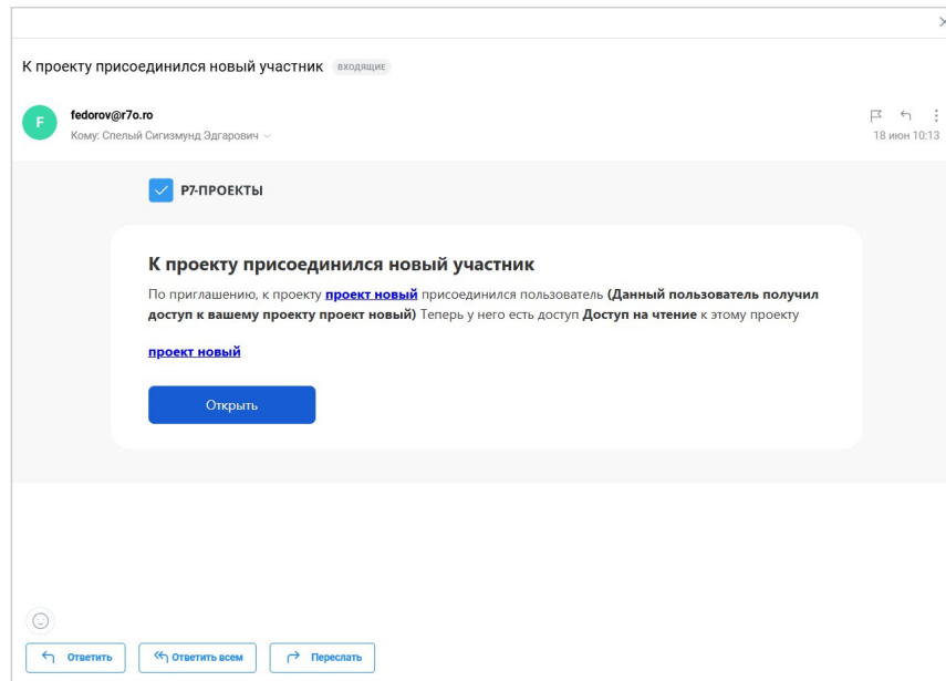
Рисунок 54 – Окно письма
