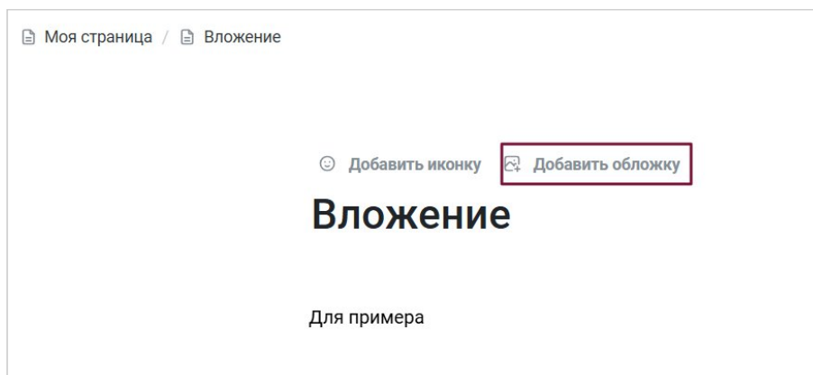
Рисунок 131 – Добавить обложку
