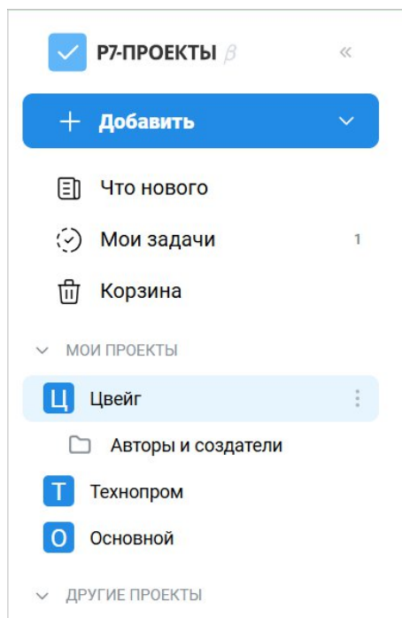
Рисунок 97 – Боковая панель
