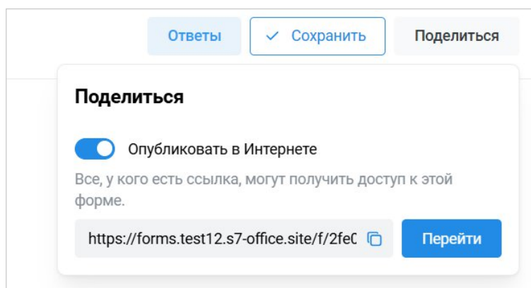
Рисунок 158 – Кнопка «Поделиться»
